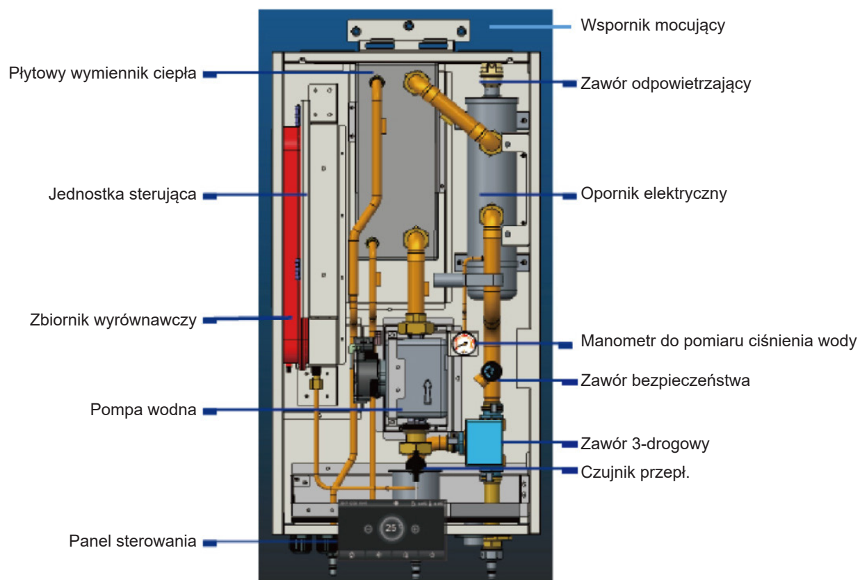
Widok wewnątrz
