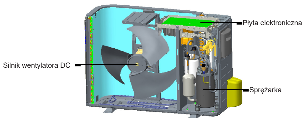
Widok wewnątrz
