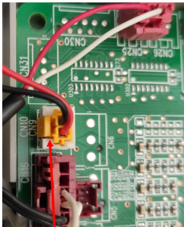
CN10 (mod.4 i 6) - CN8 (modele 8 i 10) - Czujnik temperatury zbiornika zasobnikowego
