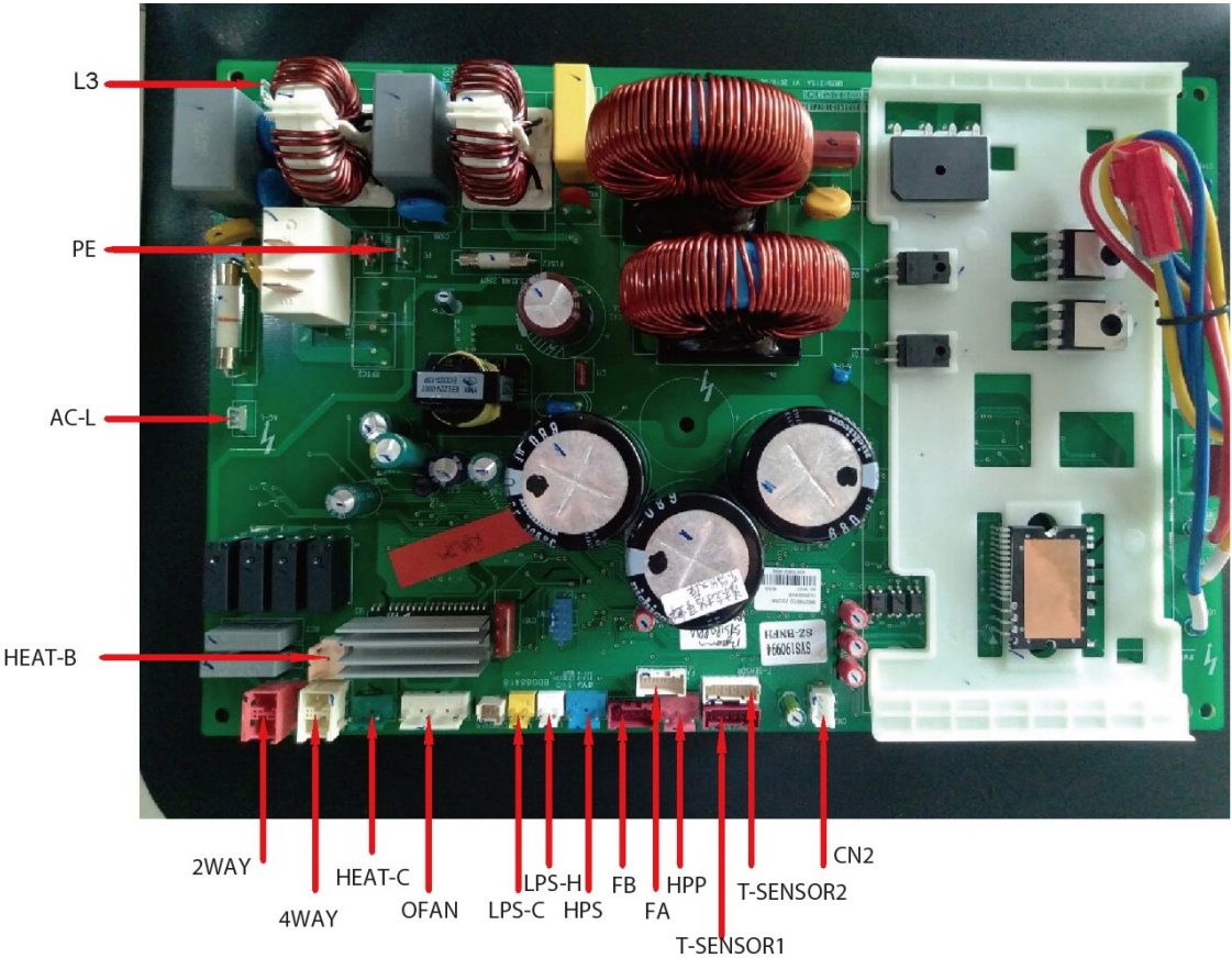
(2) Płyta jednostki zewnętrznej PROCIDA AWS 4 (O), PROCIDA AWS 6 (O)
