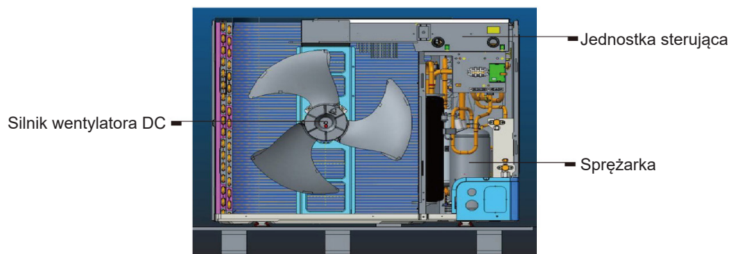
Widok wewnątrz
