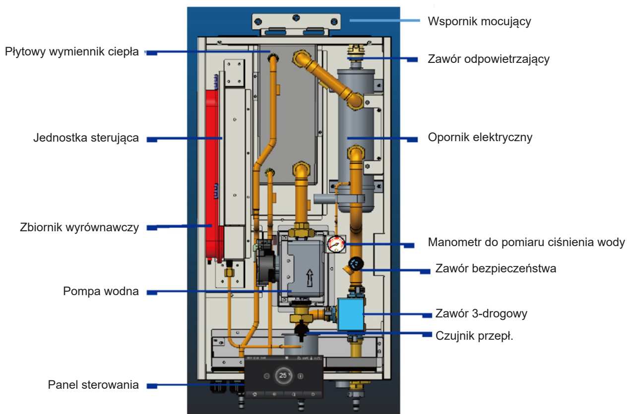
Widok wewnątrz
