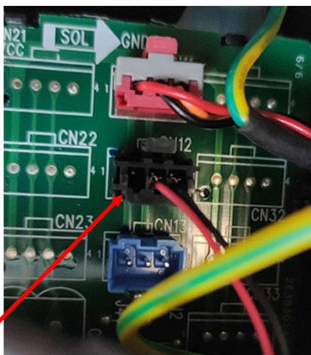
CN12-komunikacja z jednostką zewnętrzną (z CN3)
