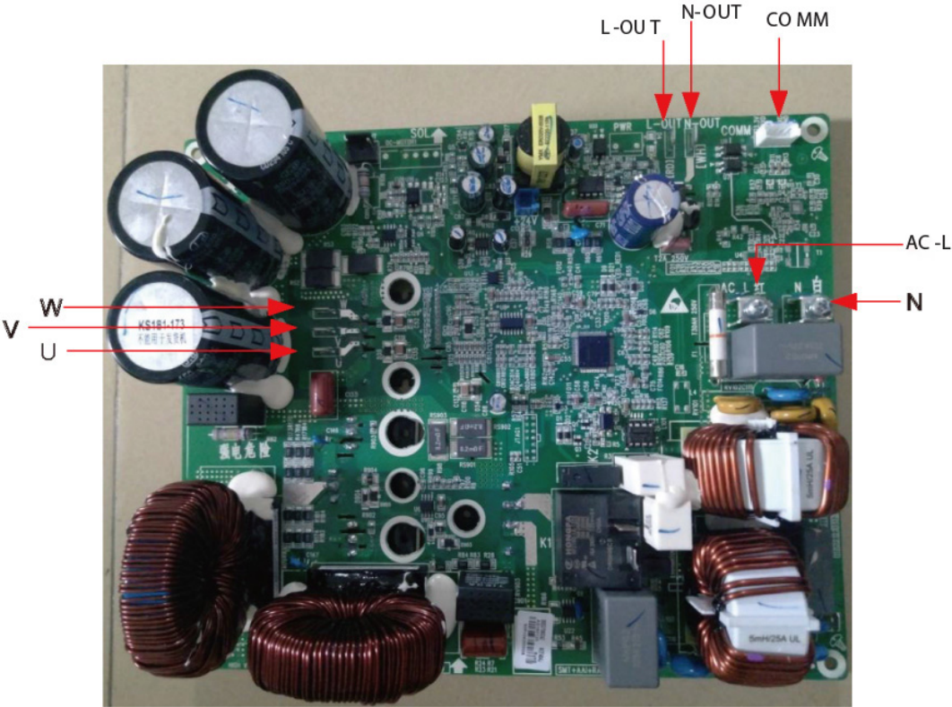
Jednostka zewnętrzna
