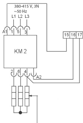
Опціональний електронагрівач 2
