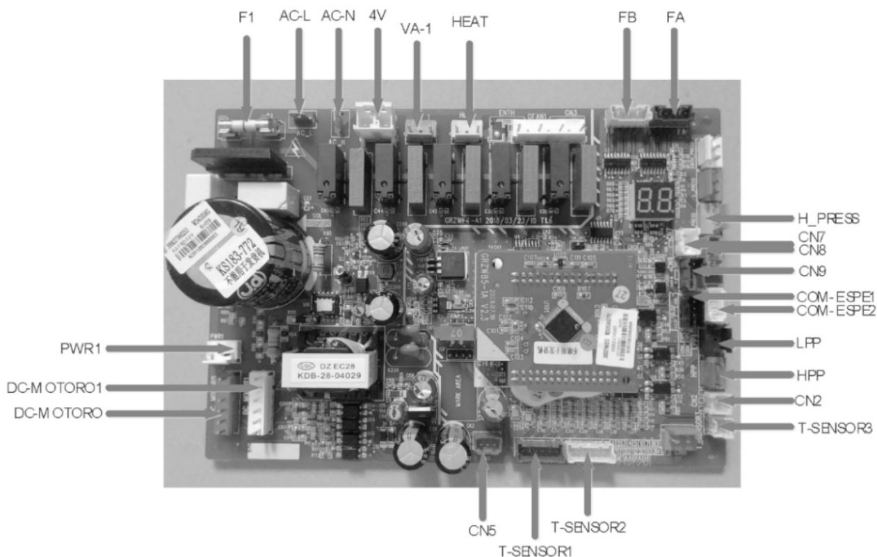
Плата AP2
