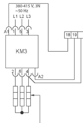
Електронагрівач бойлера
