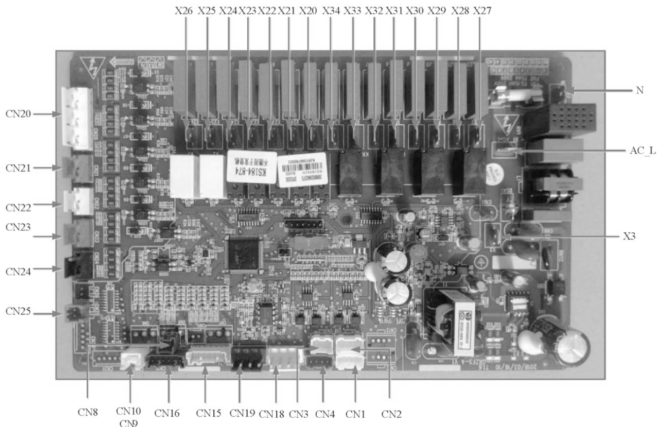
Плата AP1
