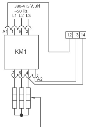
Опціональний електронагрівач 1
