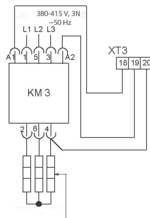
Електронагрівач бойлера
