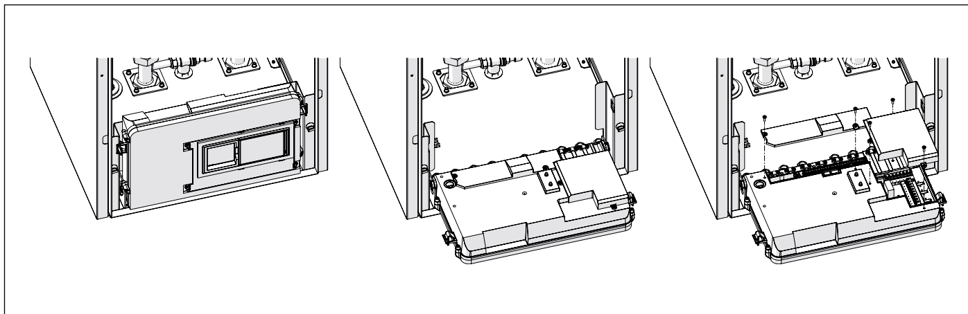
Obr. 25 Elektrická krabice
