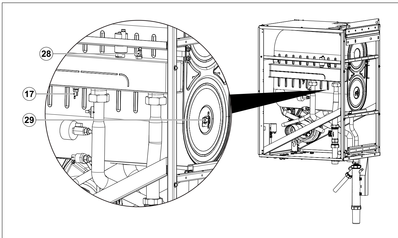
Obr. 5 Součásti (II)
