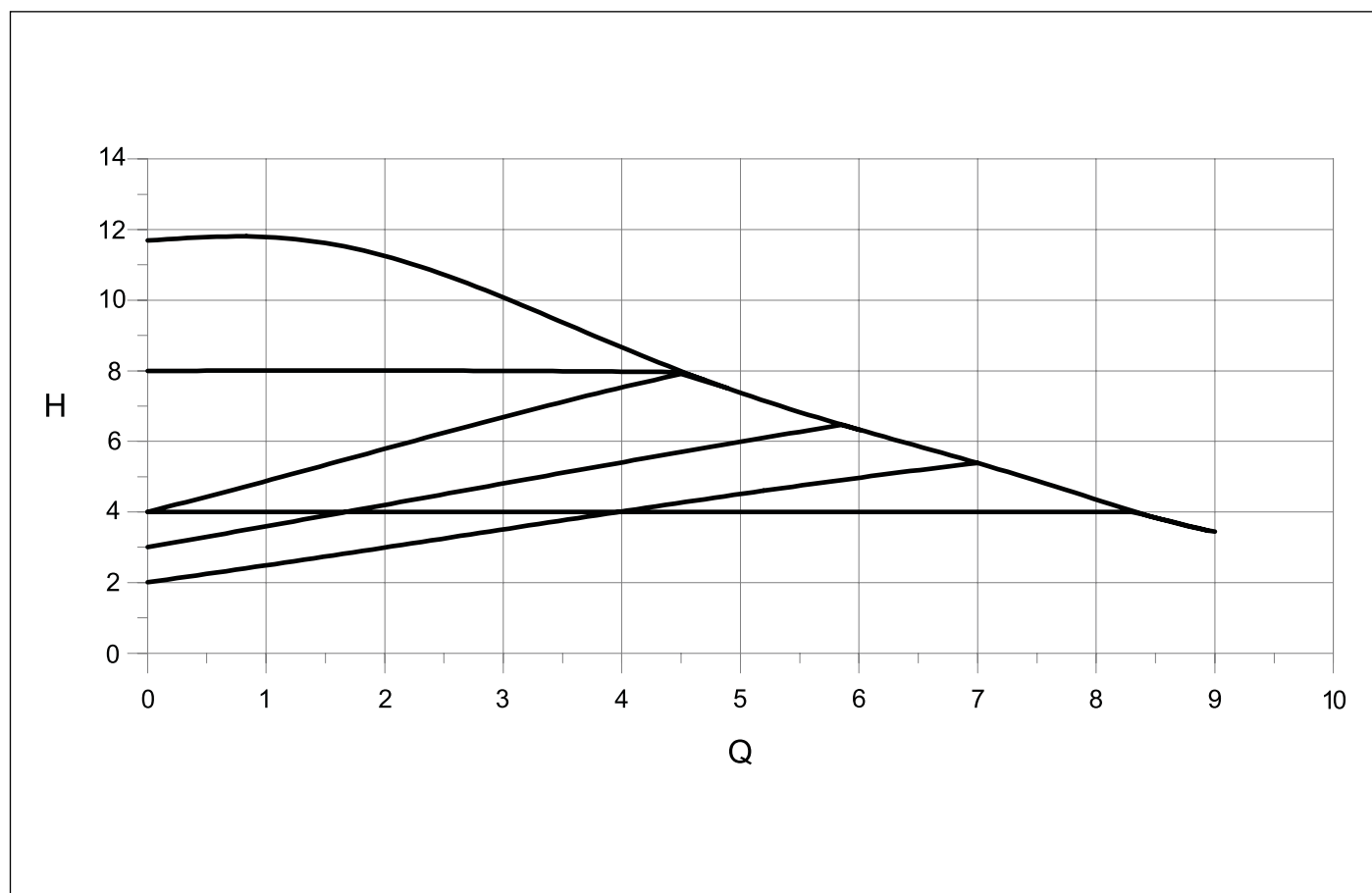
Obr. 22 Dostupná hlava UPMXXL 25 - 120 - 180 AUTO
