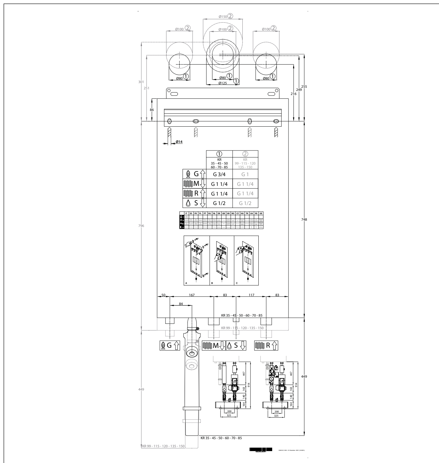
Obr. 7 Papírová šablona
