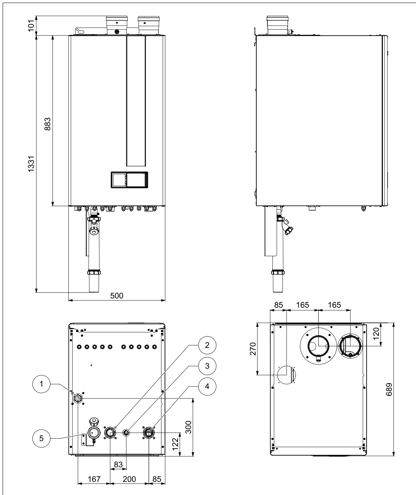
Obr. 3 Rozměry
