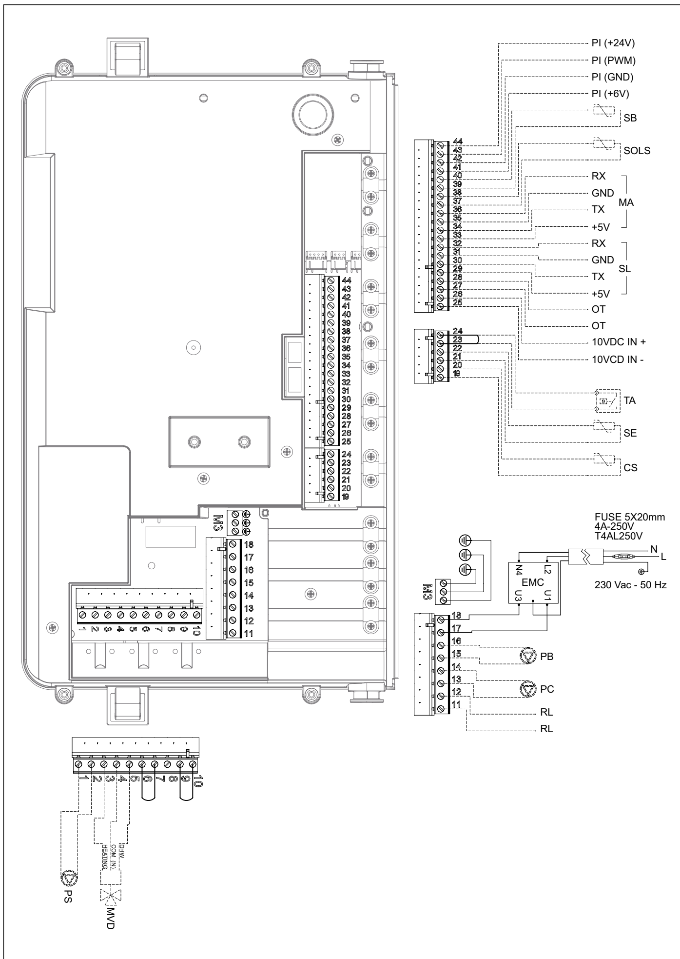
Obr. 27 Připojení, která provede instalatér
