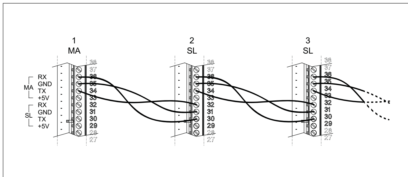
Obr. 28 Kaskádové připojení
