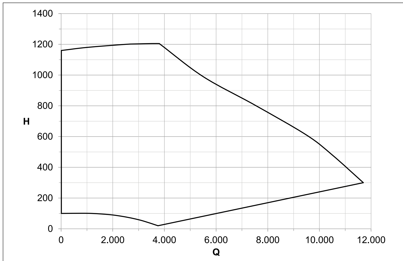
Obr. 20 Dostupná hlava YONOS PARA HF 25/12
