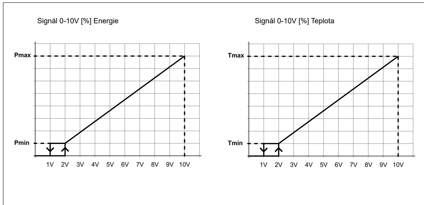
Obr. 18 Signál 0-10VDC
