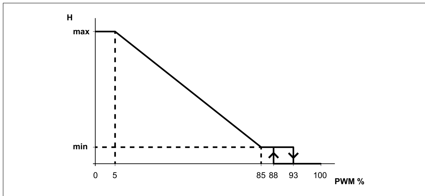
Obr. 23 Signál PWM
