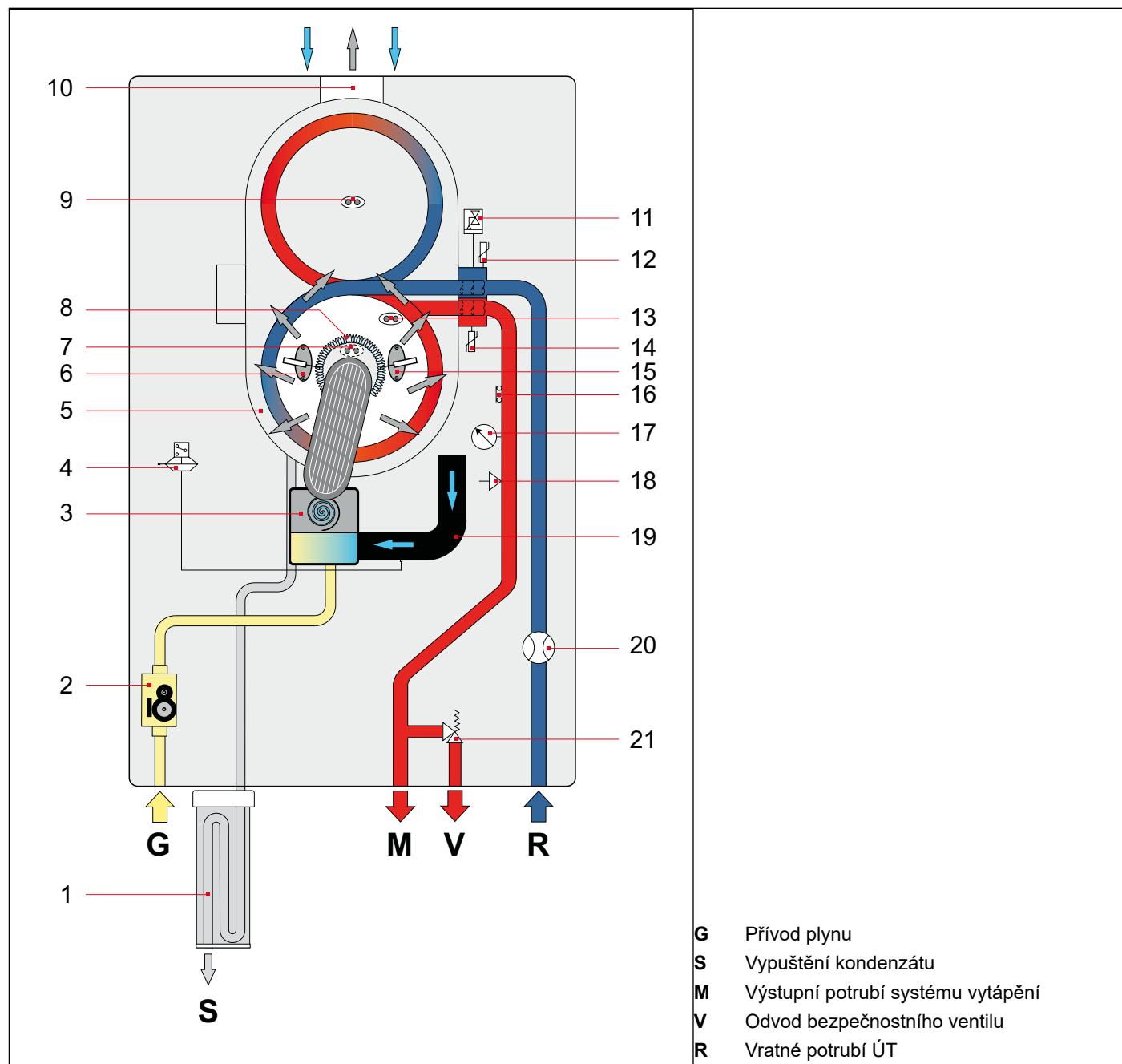
Obr. 6 Uspořádání kotle
