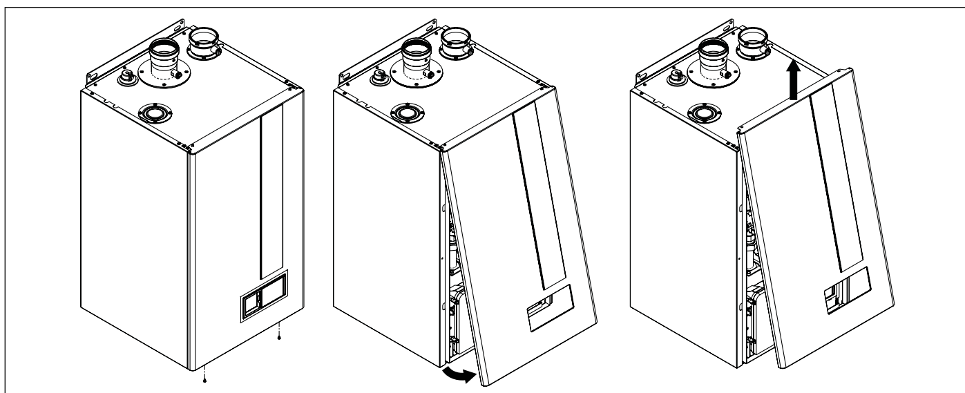
Obr. 29 Otvírání pláště
