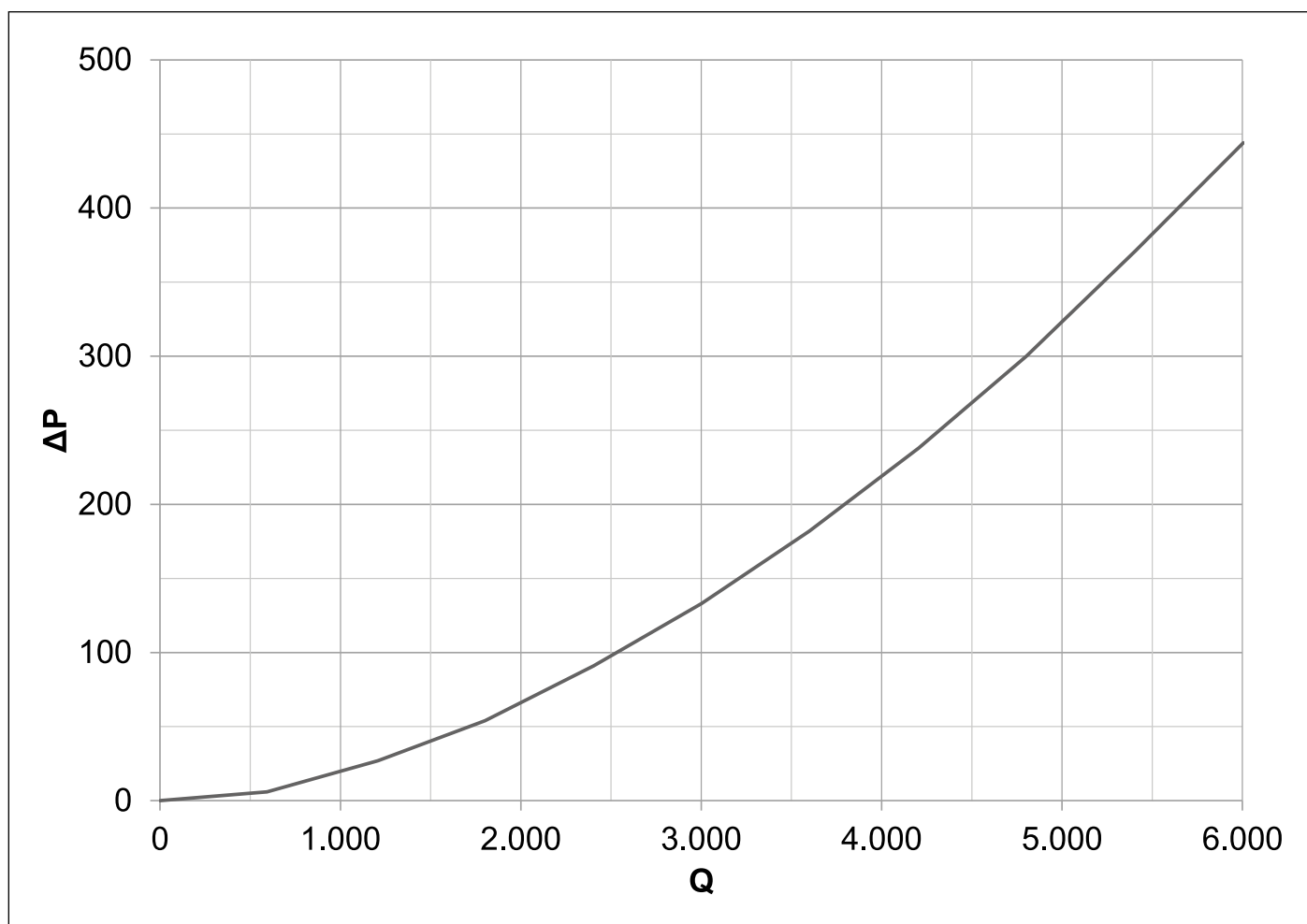
Obr. 19 Hydraulický odpor
