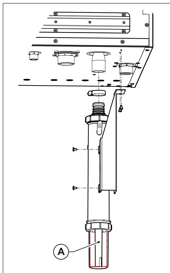
Obr. 8 Připevnění sifonu
