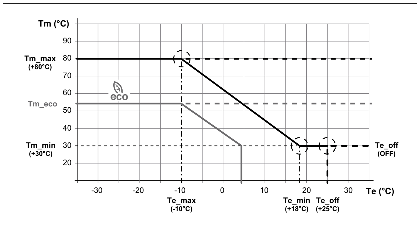
Obr. 17 Klimatická křivka
