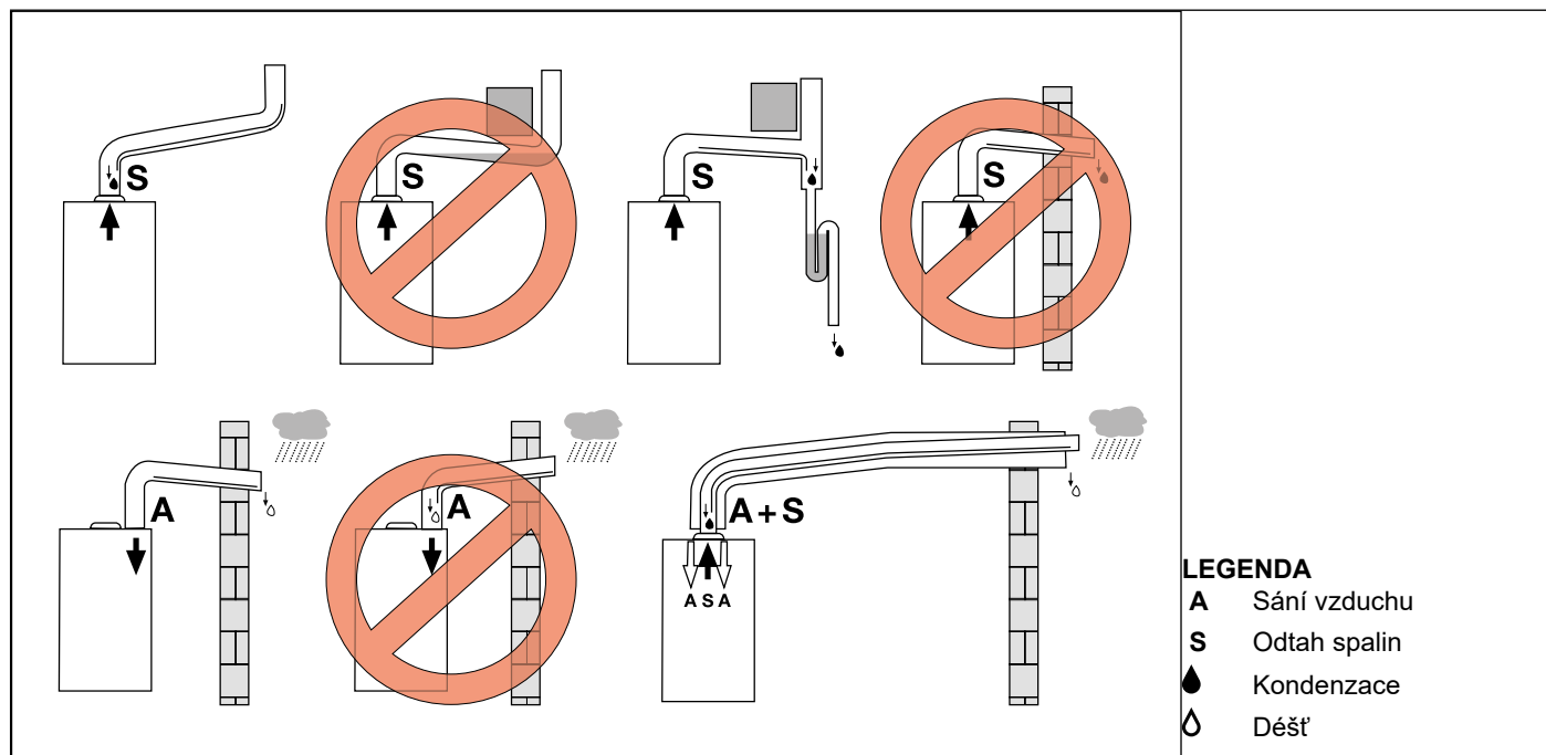
Obr. 11 Příklad instalace
