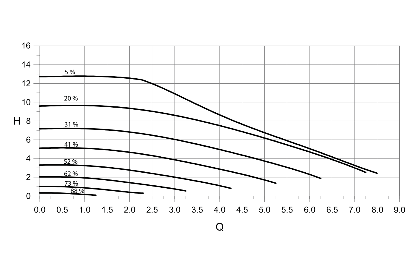
Obr. 21 Dostupná hlava UPMXL 25 - 125 - 180 PWM
