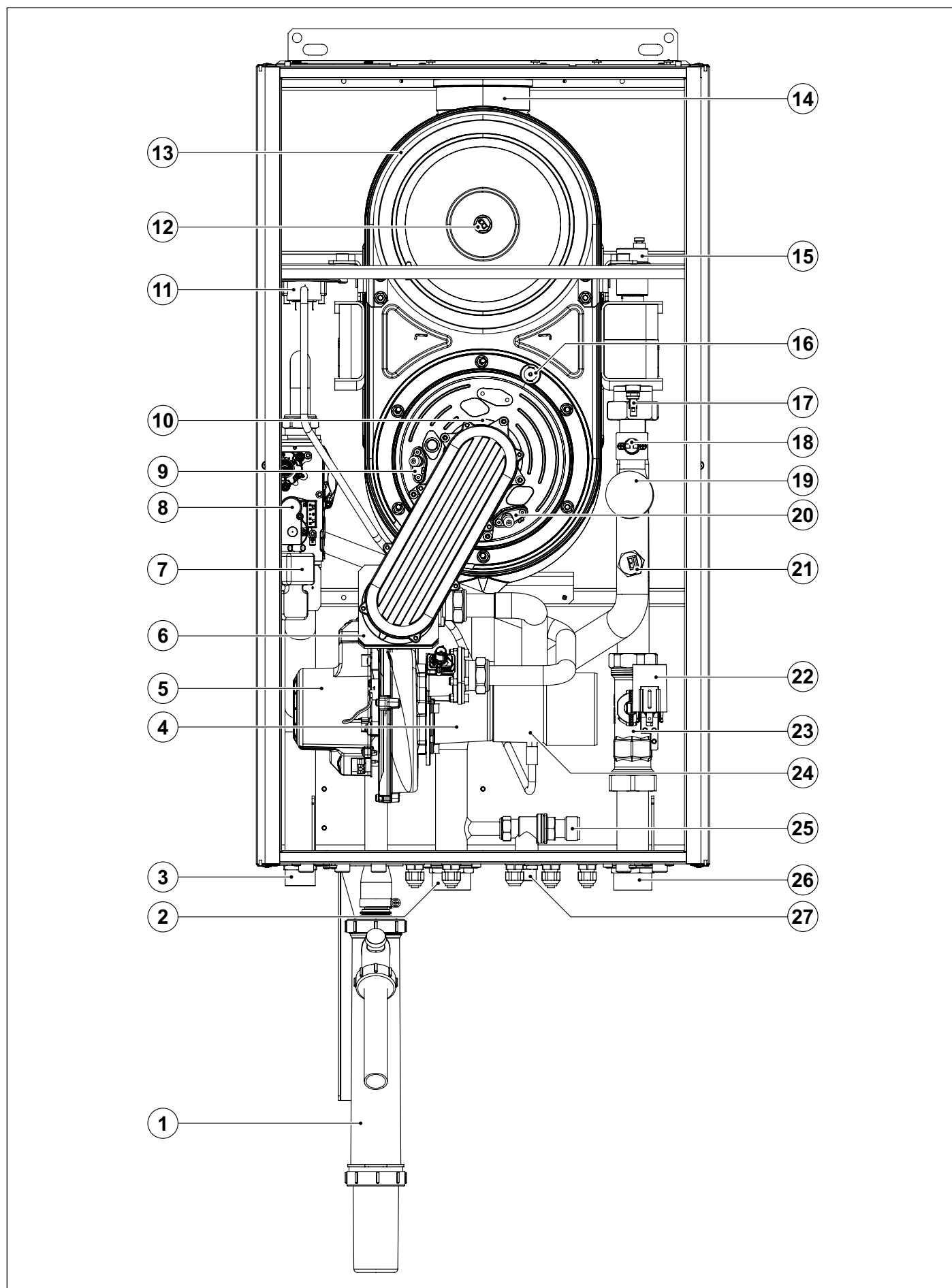
Obr. 4 Součásti (I)
