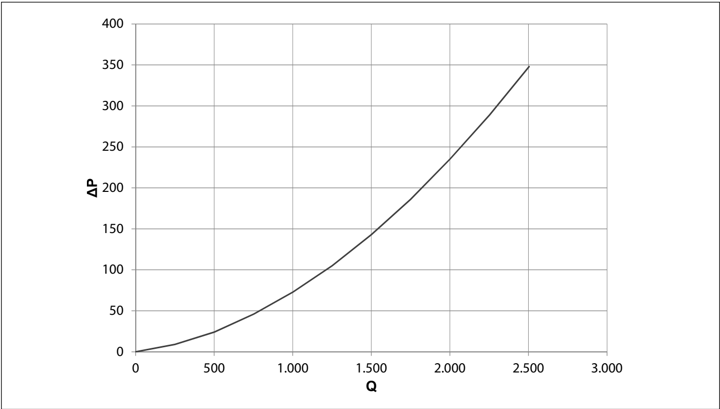
Fig. 22 Resistencia hidráulica KR 60
