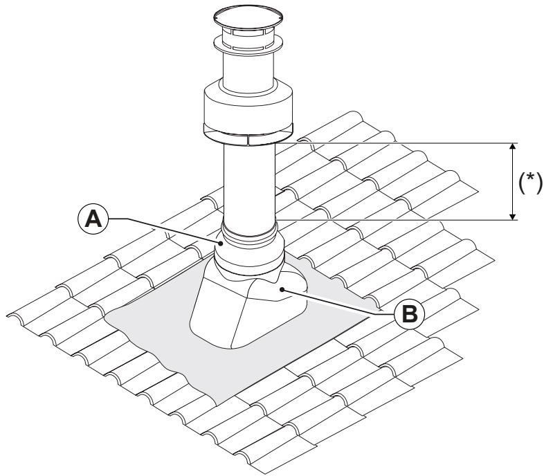
Fig. 17 Instalación chimenea en el tejado
