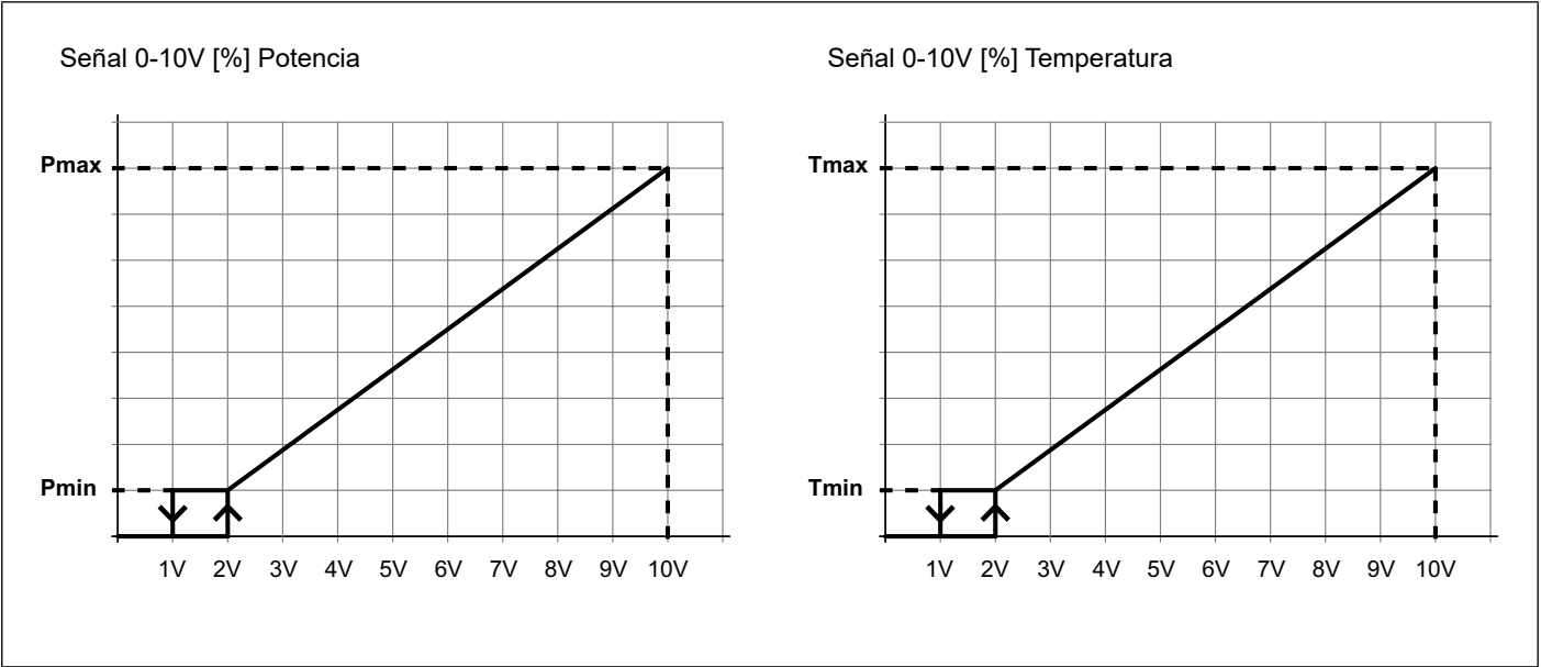
Fig. 20 Señal 0-10VDC
