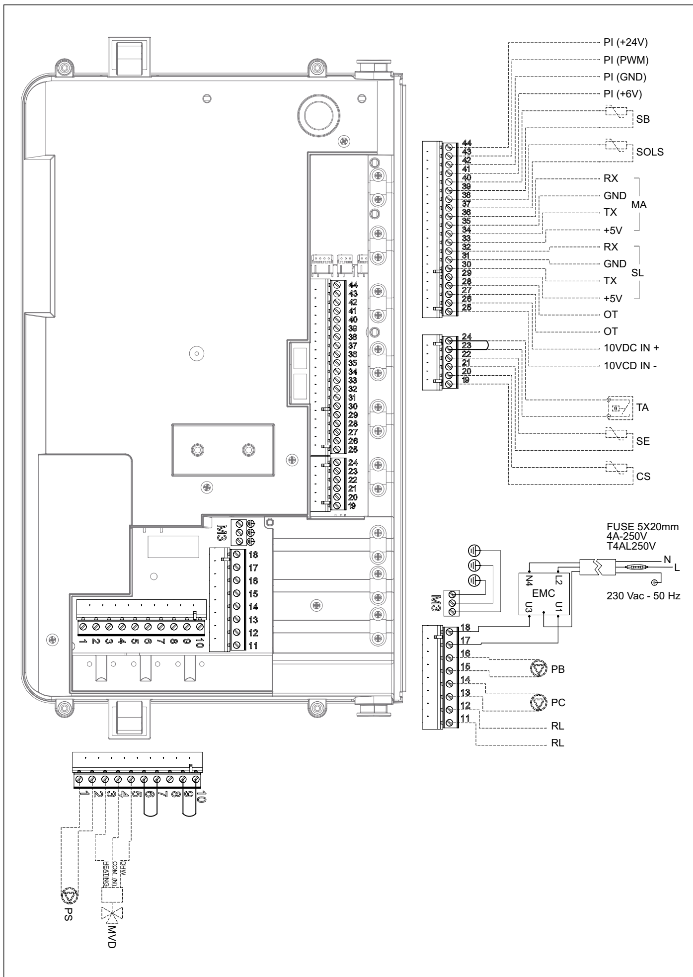
Fig. 29 Conexiones a cargo del instalador
