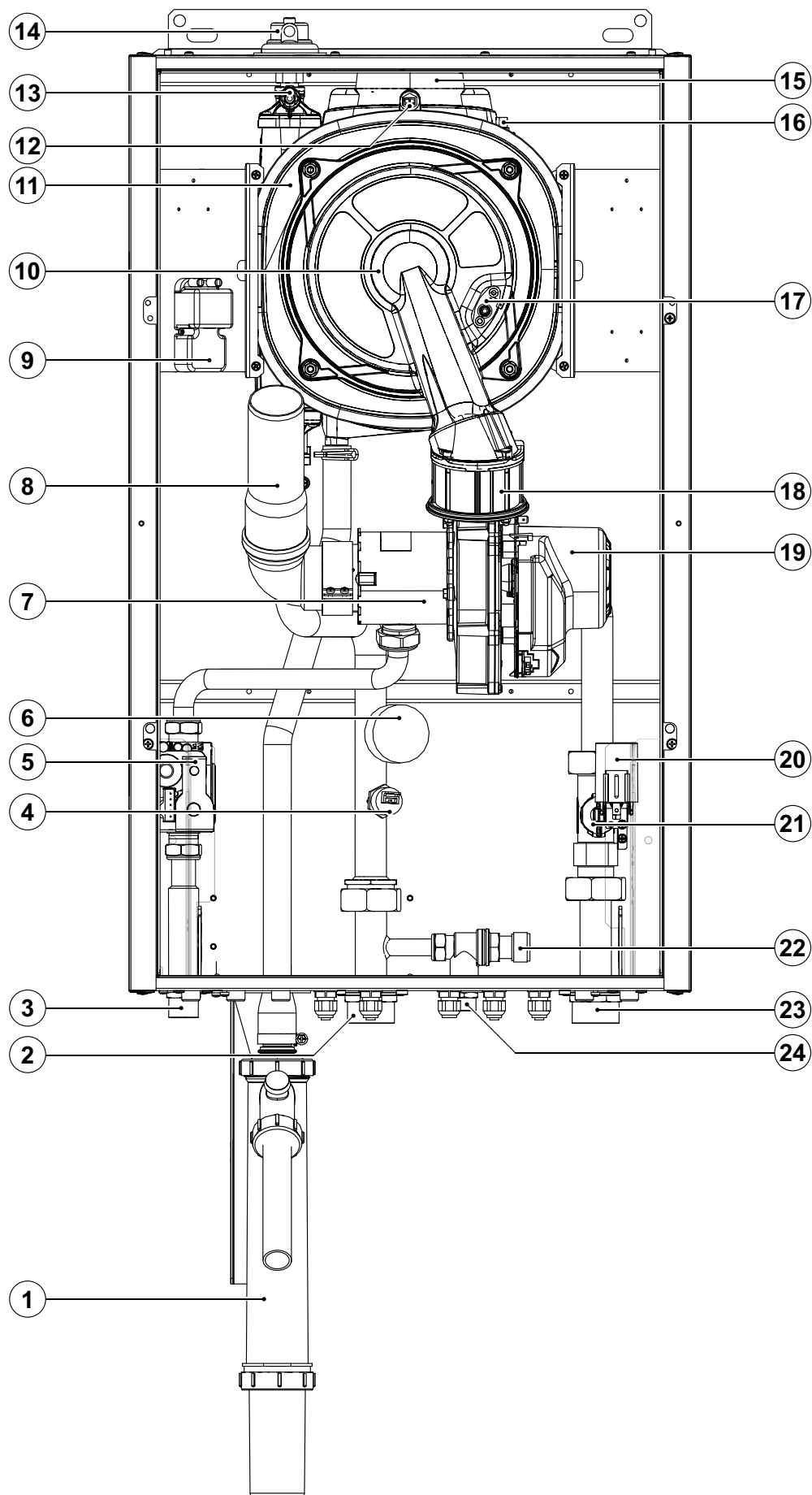
Fig. 6 Componentes KR 60 (I)
