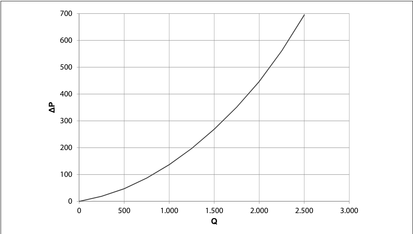
Fig. 21 Resistencia hidráulica KR 45
