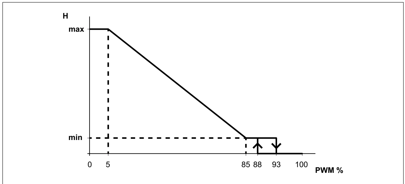
Fig. 33 Semnal PWM
