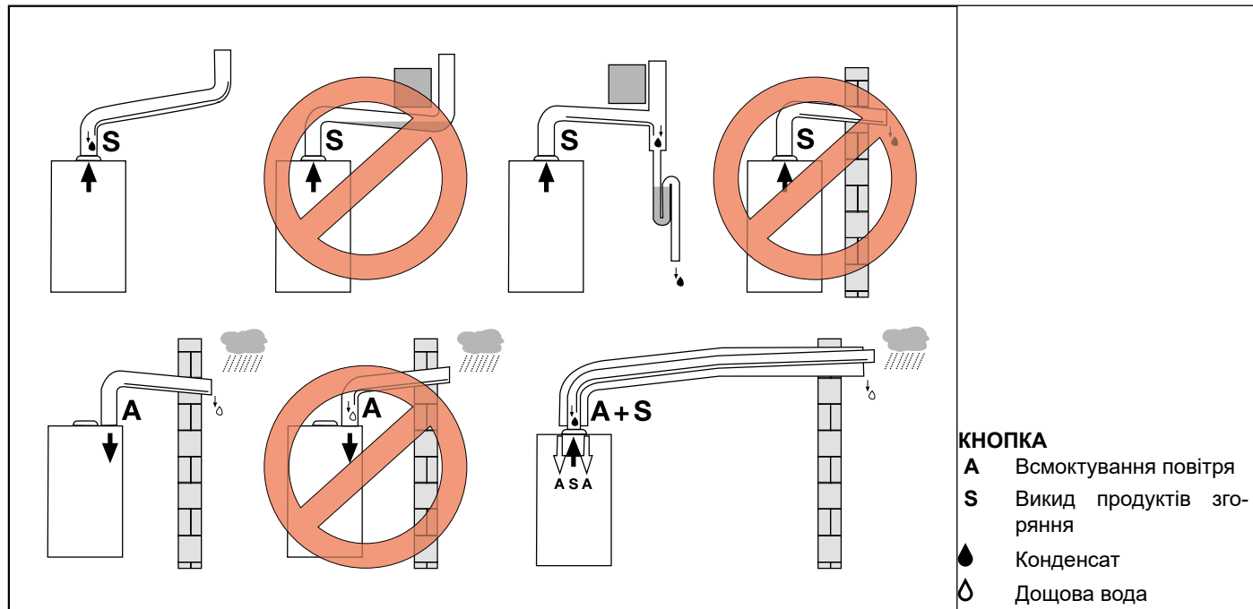
Рис. 13 Приклади монтажу
