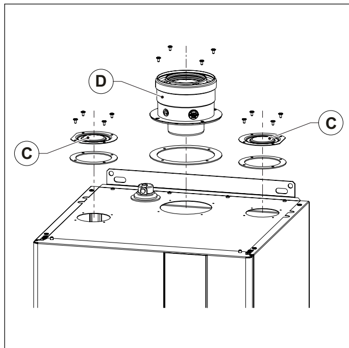
Рис. 12 Установка коаксіального набору
