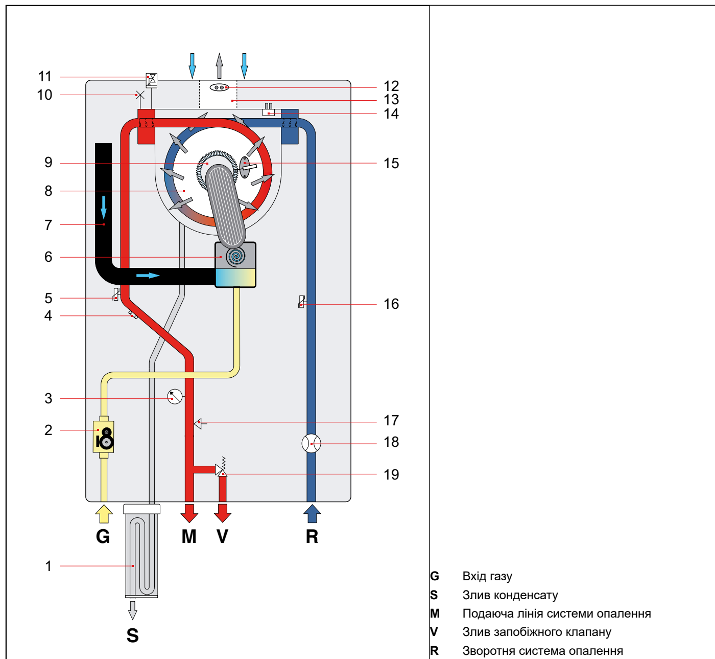
Рис. 8 Схеми гідравлічних підключень KR 45 - KR 60
