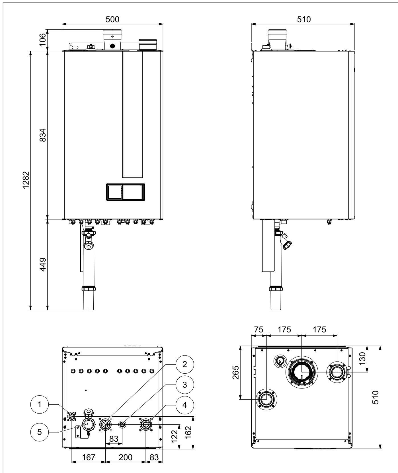
Рис. 3 Габарити KR 45 - KR 60
