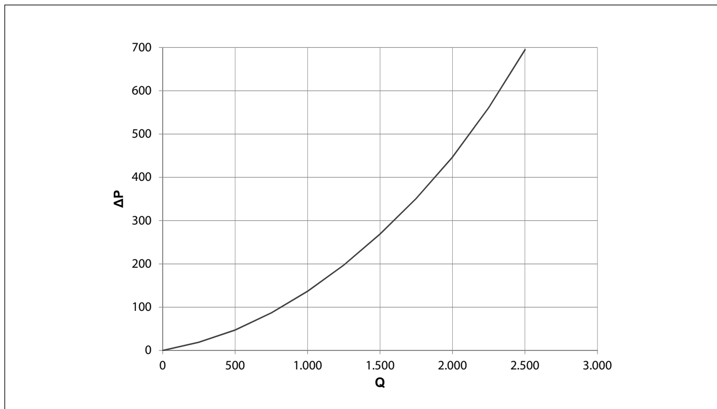
Рис. 21 Гідравлічний опір KR 45
