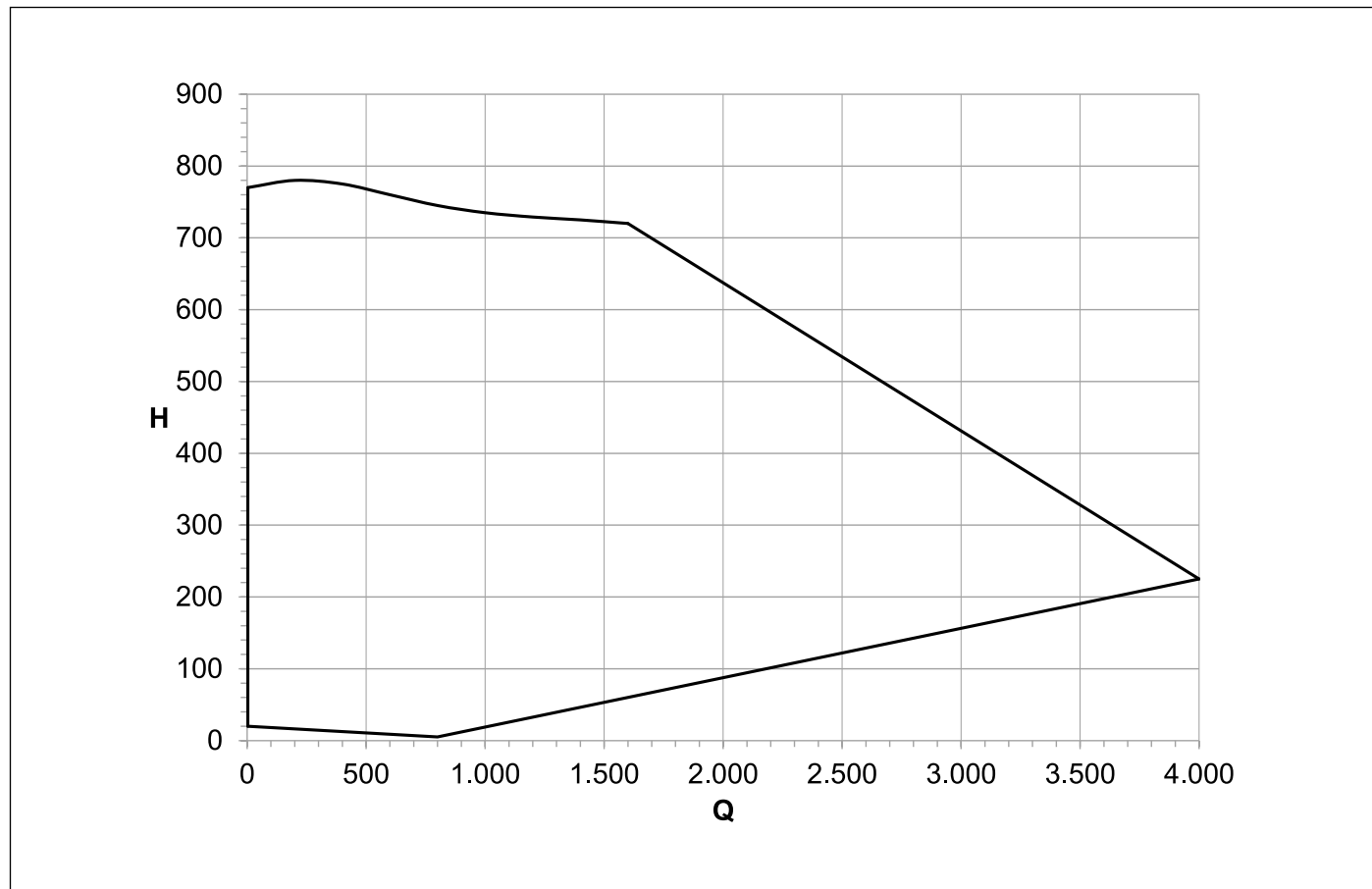
Рис. 23 Наявний напір YONOS PARA RS 25/7.5
