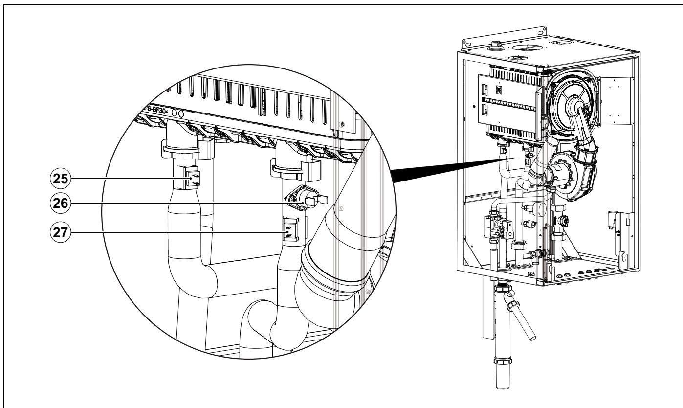
Рис. 7 Компоненти KR 60 (II)
