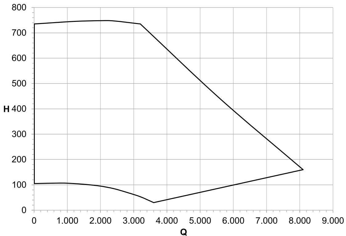
Рис. 24 Наявний напір YONOS PARA HF 25/7
