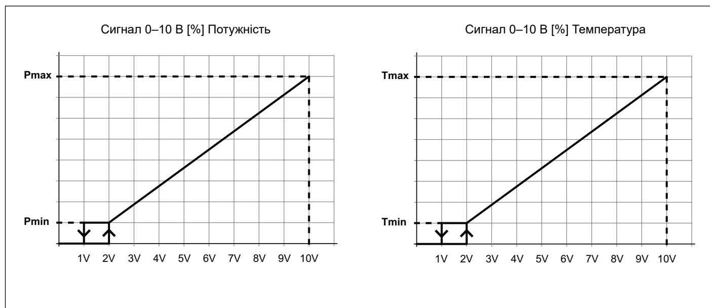
Рис. 20 Сигнал 0–10 В постійного струму
