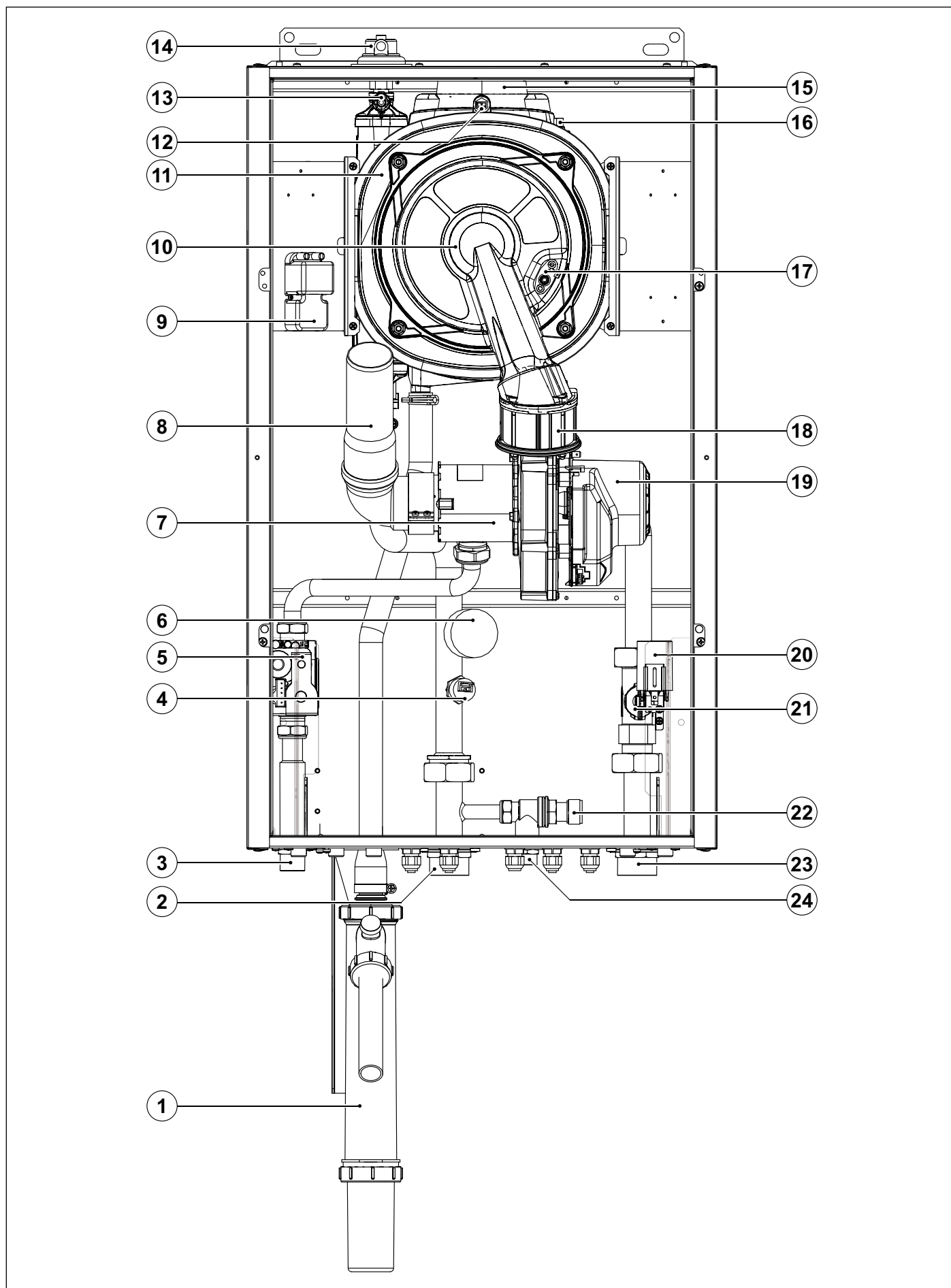
Рис. 6 Компоненти KR 60 (I)
