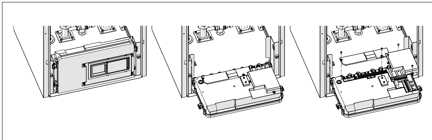
Рис. 27 Блок електрики
