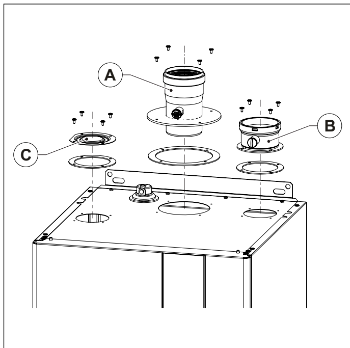
Рис. 11 Установка розгалуженого набору
