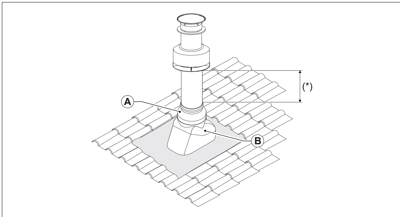
Рис. 17 Установка дымоходу на даху
