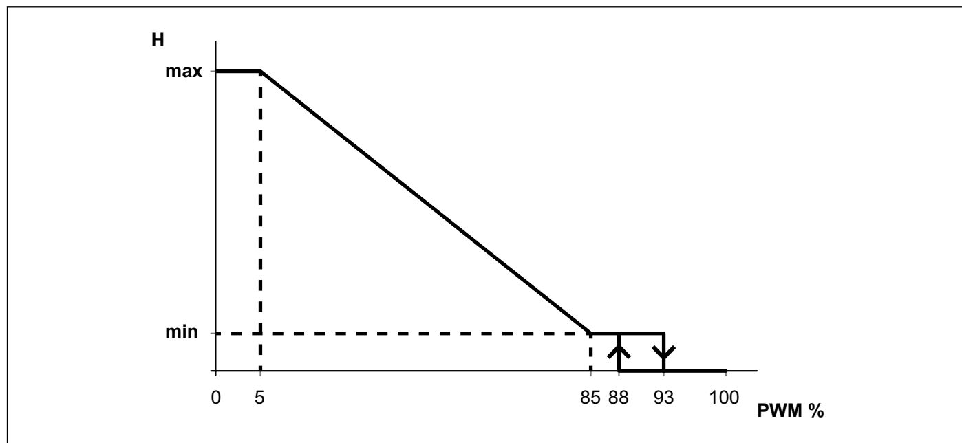
Рис. 25 Сигнал ШІМ
