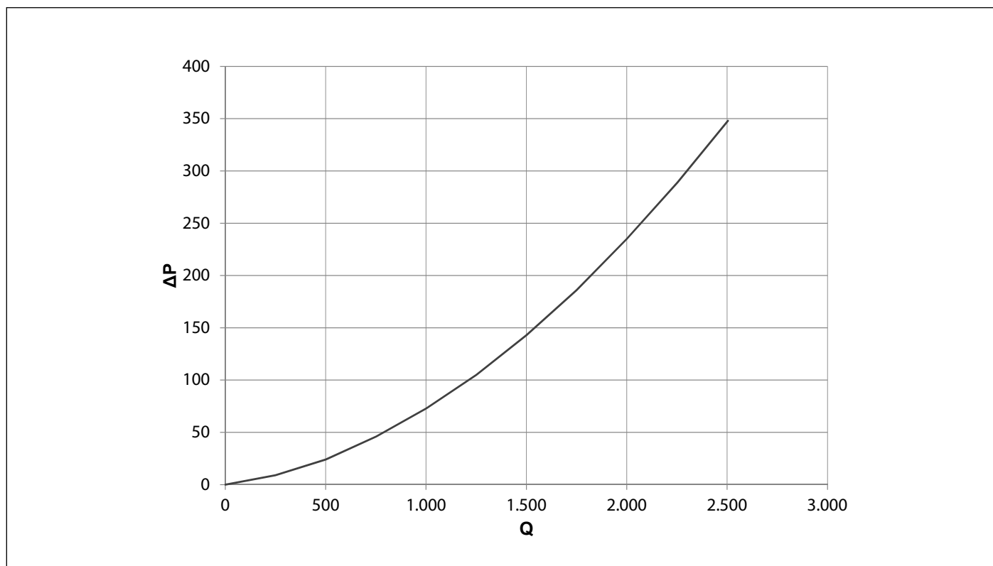
Рис. 22 Гідравлічний опір KR 60
