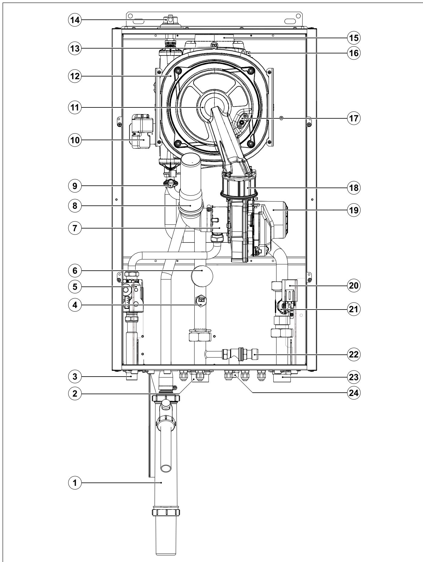
Рис. 4 Компоненти KR 45 (I)
