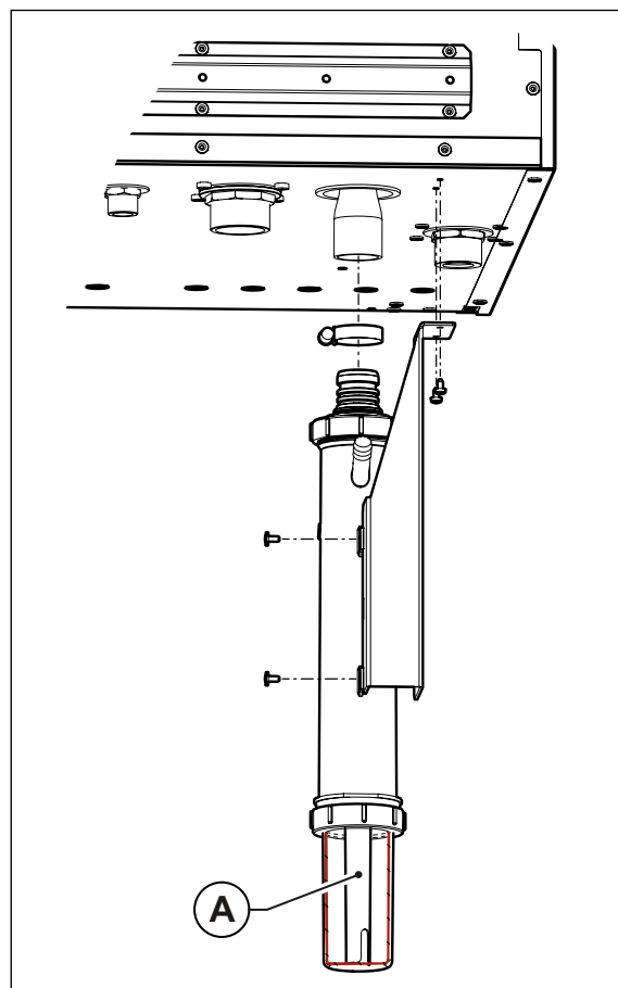
Рис. 10 Закріплення збірника
