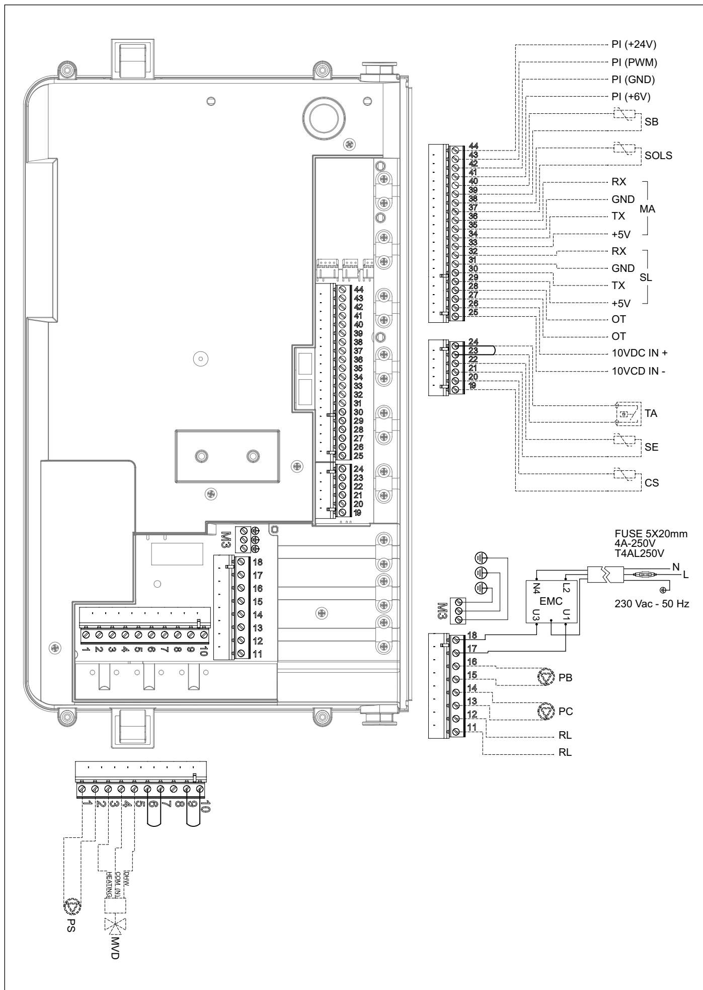
Рис. 29 Усі підключення виконуються монтажником
