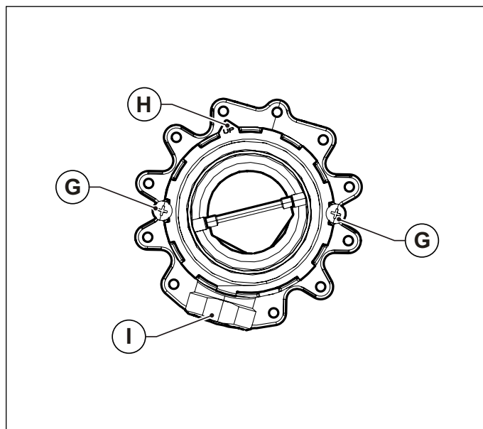
Рис. 35 Розташування для монтажу
