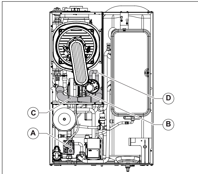
Obr. 32 Sací trubice
