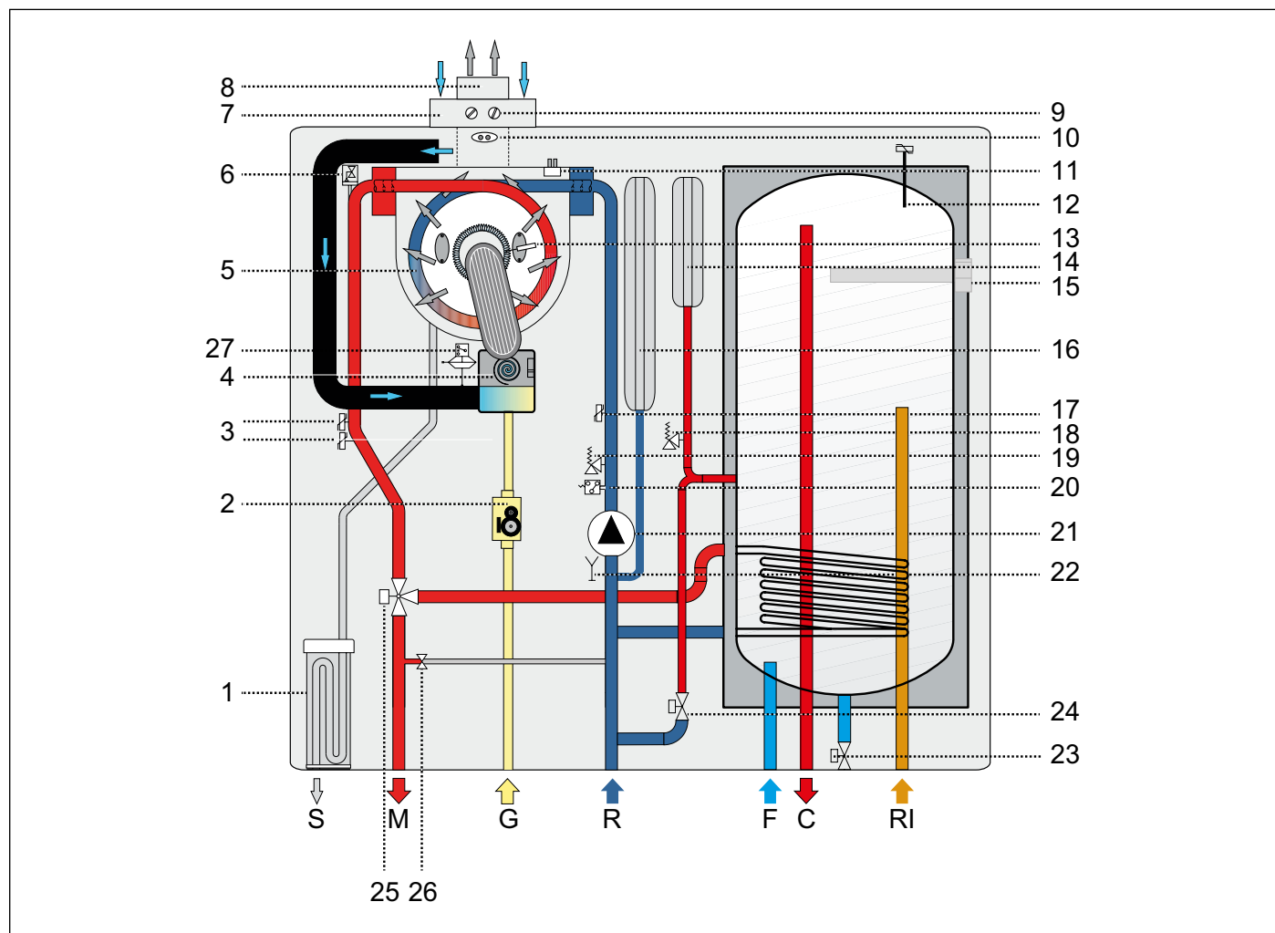
Obr. 5 Uspořádání kotle
