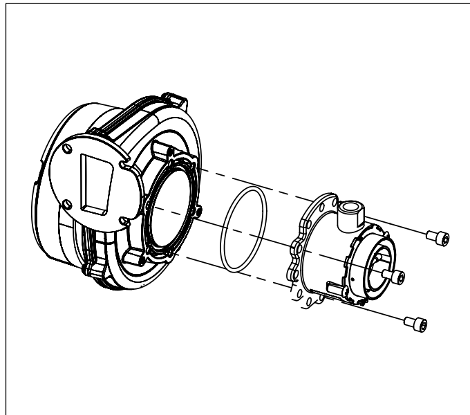
Obr. 33 Směšovač
