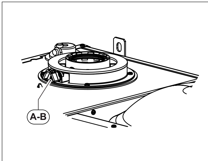
Obr. 19 Pozice uzávěrů
