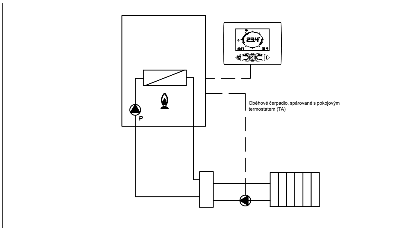
Obr. 29 Relé spuštěné dálkovým ovladačem (P17=1)
