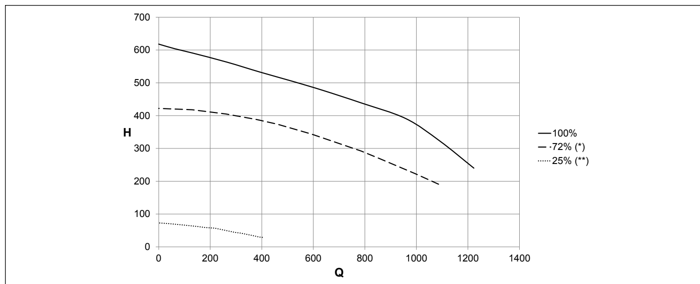
Obr. 24 Dostupná hlava KB 32
