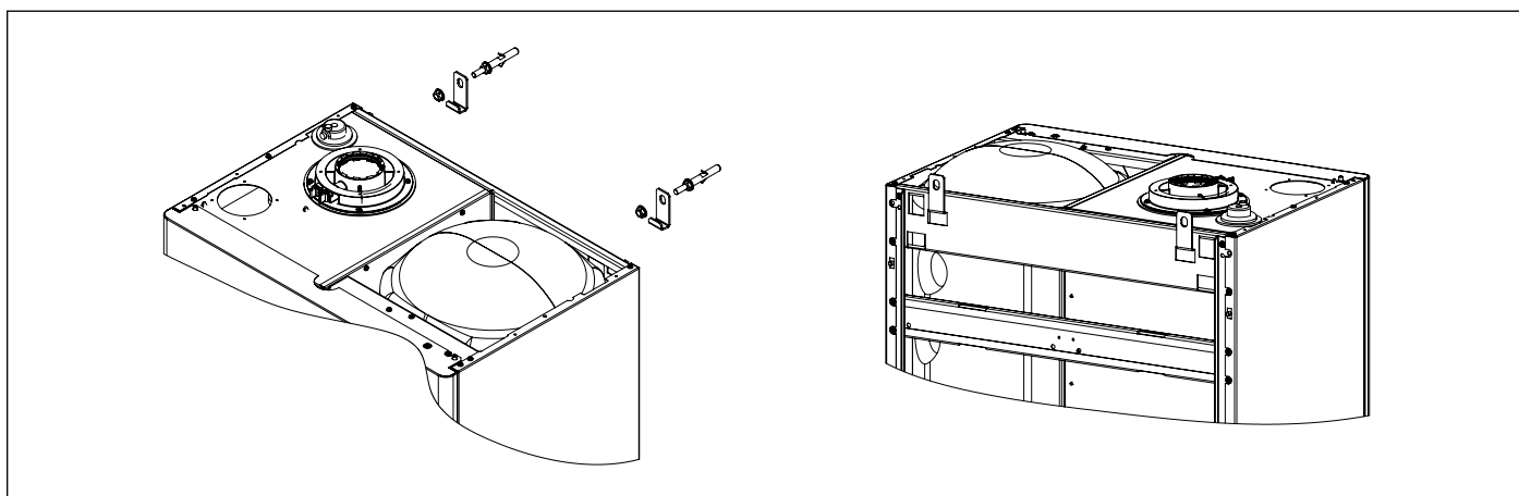
Obr. 7 Montáž podpůrných konzolí
