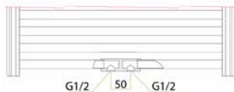
PODŁĄCZENIE ŚRODKOWE
