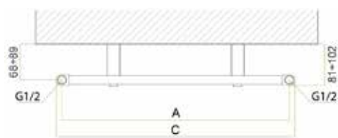
PODŁĄCZENIE BOCZNE
