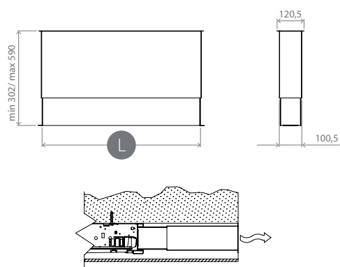
Canale di mandata telescopico per installazioni orizzontali in controsoffitto
