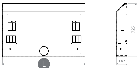
Pannello telaio installazione verticale
