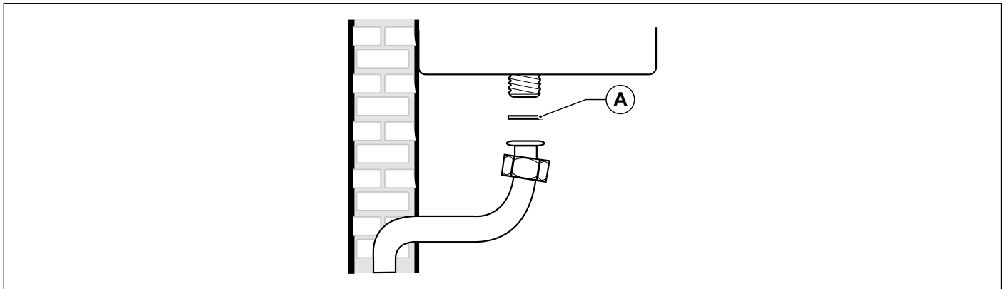
Рис. 17 Підключення газу
