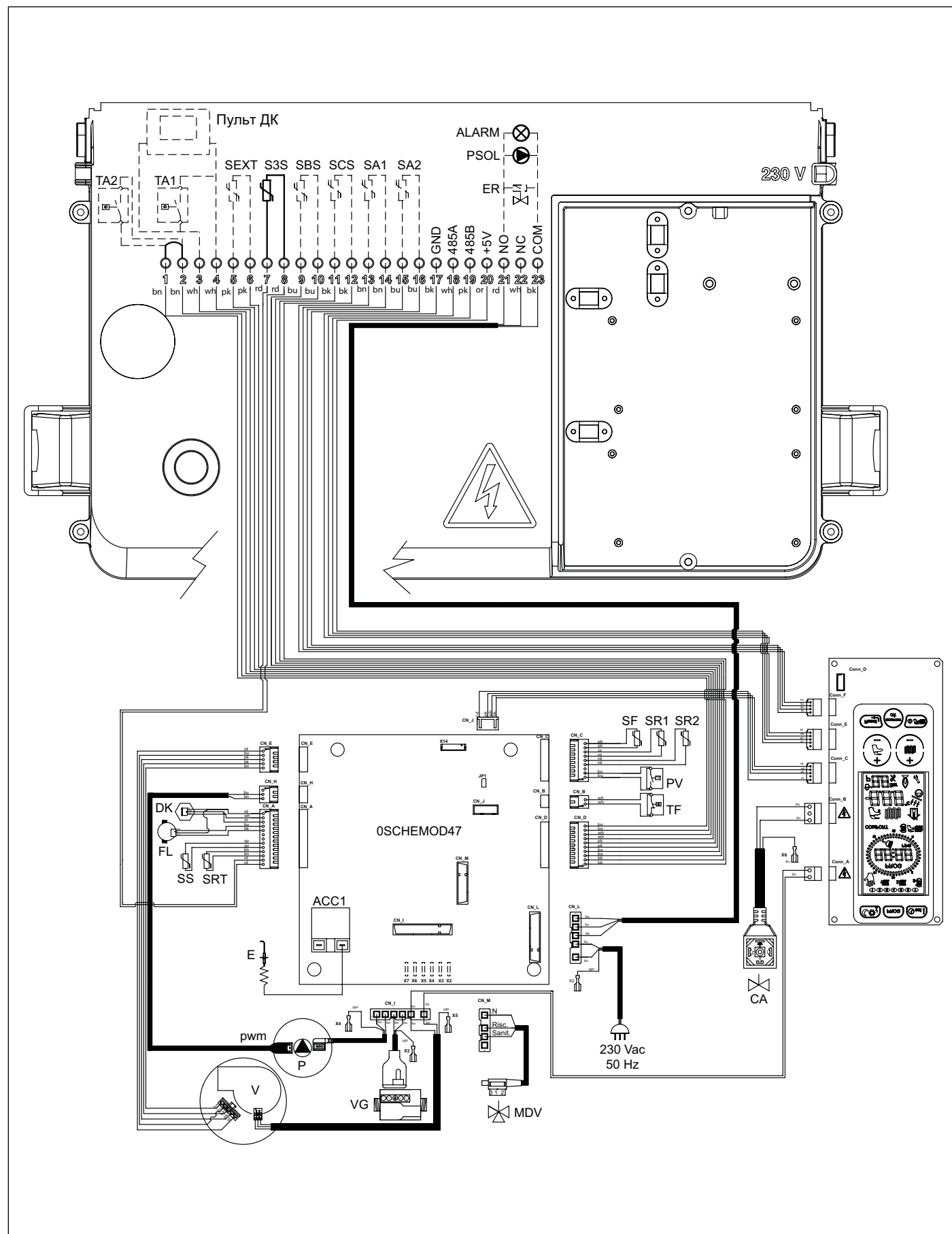
Рис. 24 Електрична схема КС
