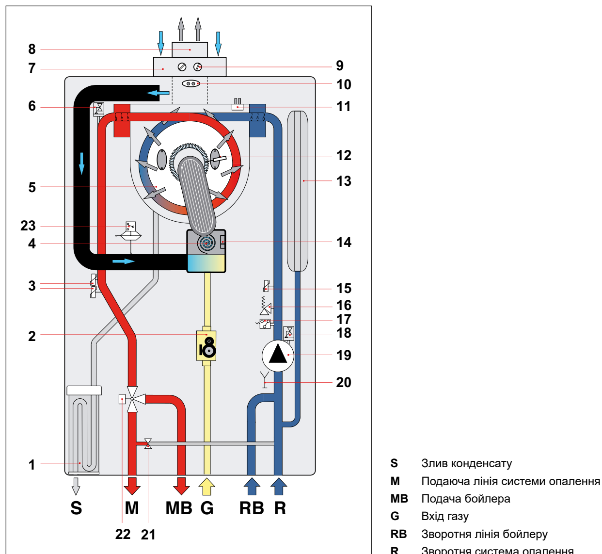
Рис. 8 Гідравлічна схема моделі KRB
