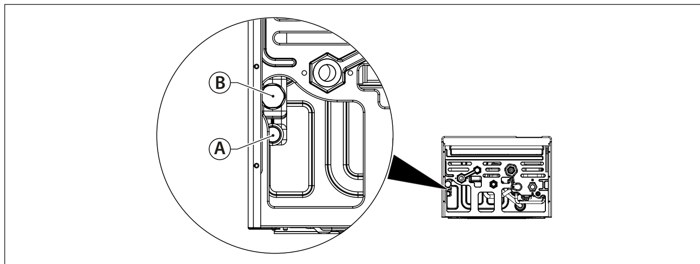
Obr. 23 Vypuštění kondenzátu
