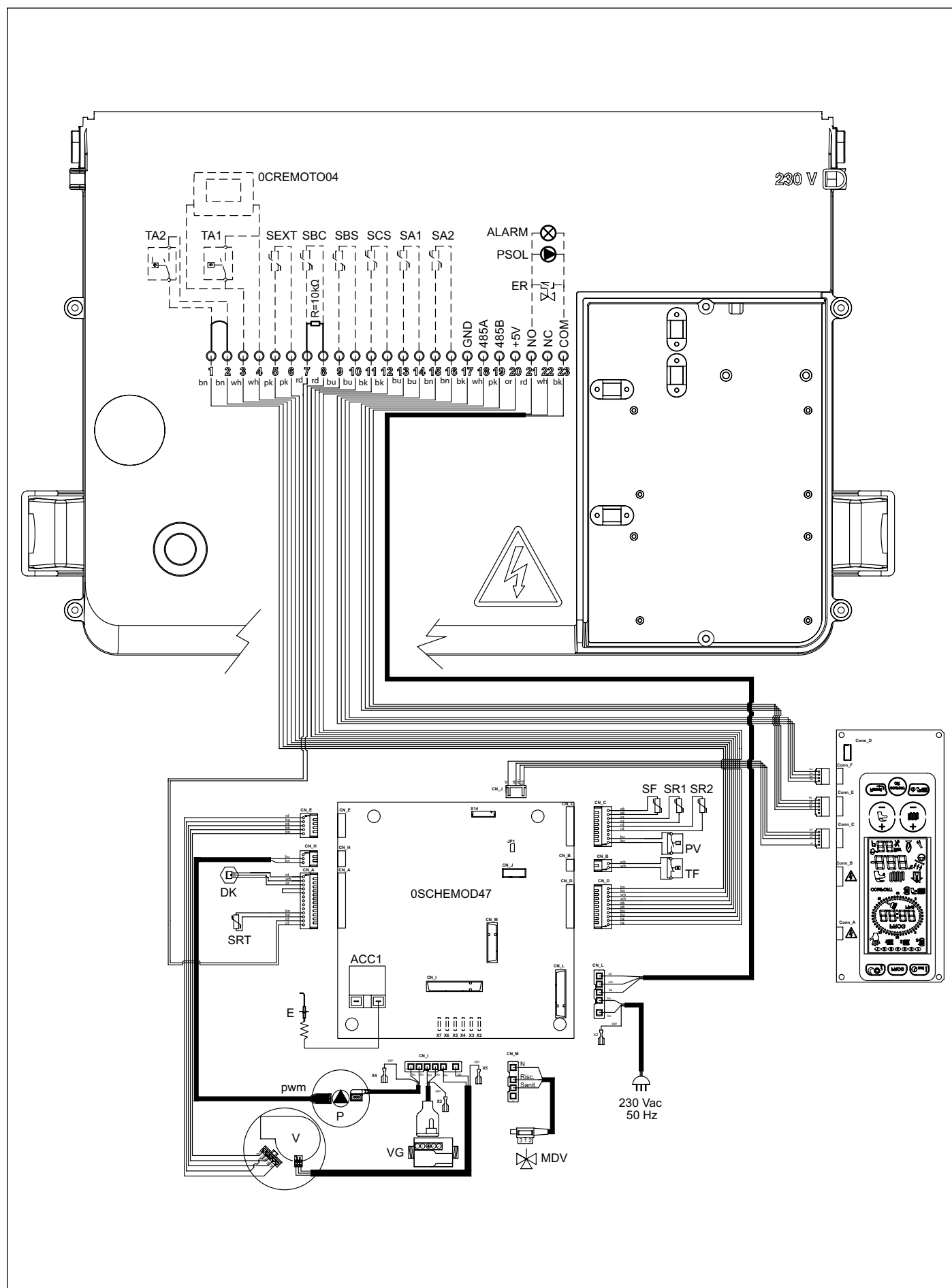
Obr. 37 Elektrické schéma KRB
