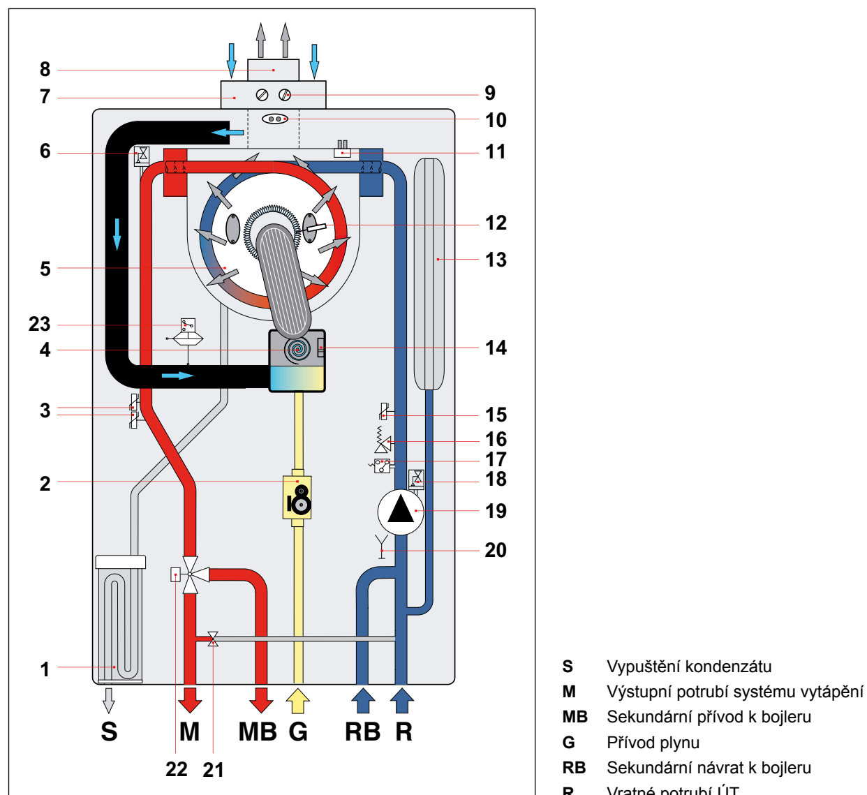
Obr. 8 Hydraulické schéma pro model KRB
