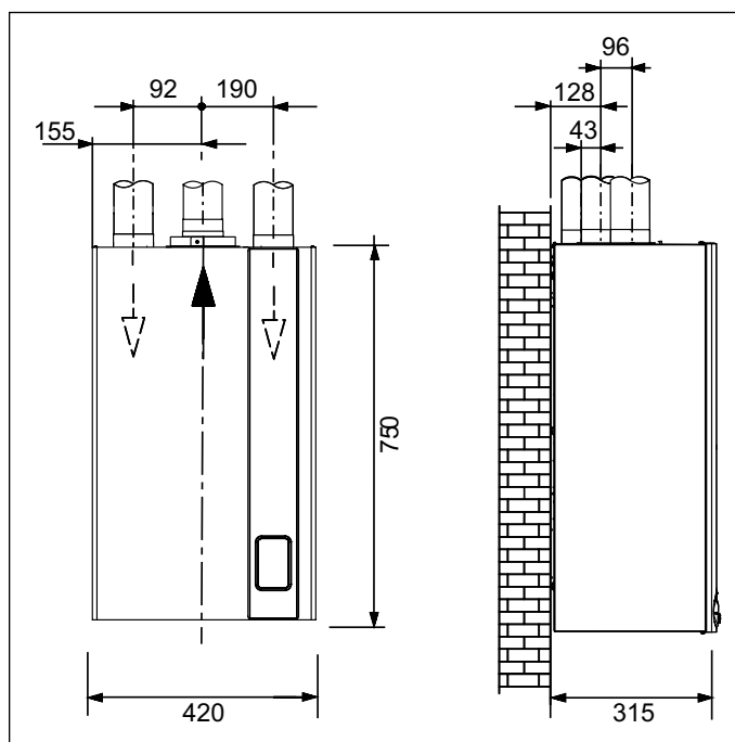
Fig. 19 Dimensiones conductos coaxiales tipo C43 - C53 - C83
