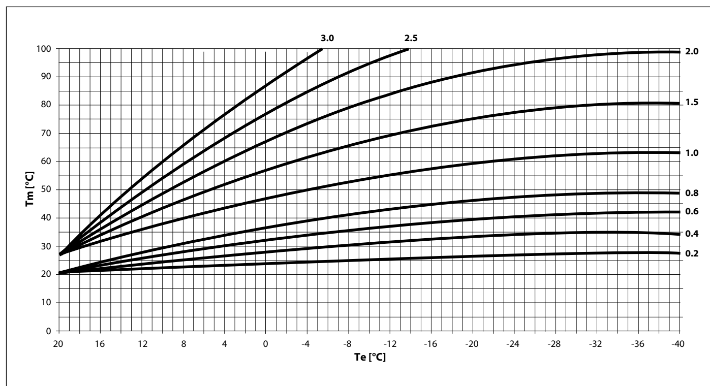
Fig. 24 Curvas de termorregulación
