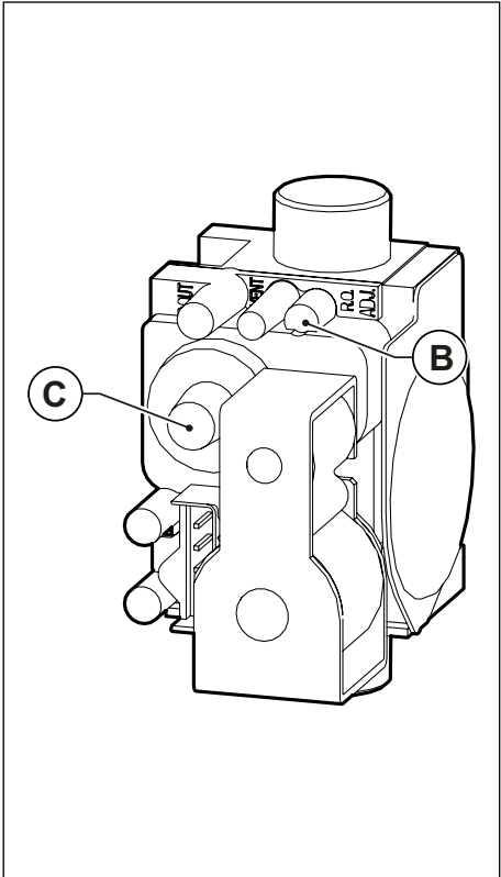
Fig. 45 Regulación valor anhídrido carbónico
