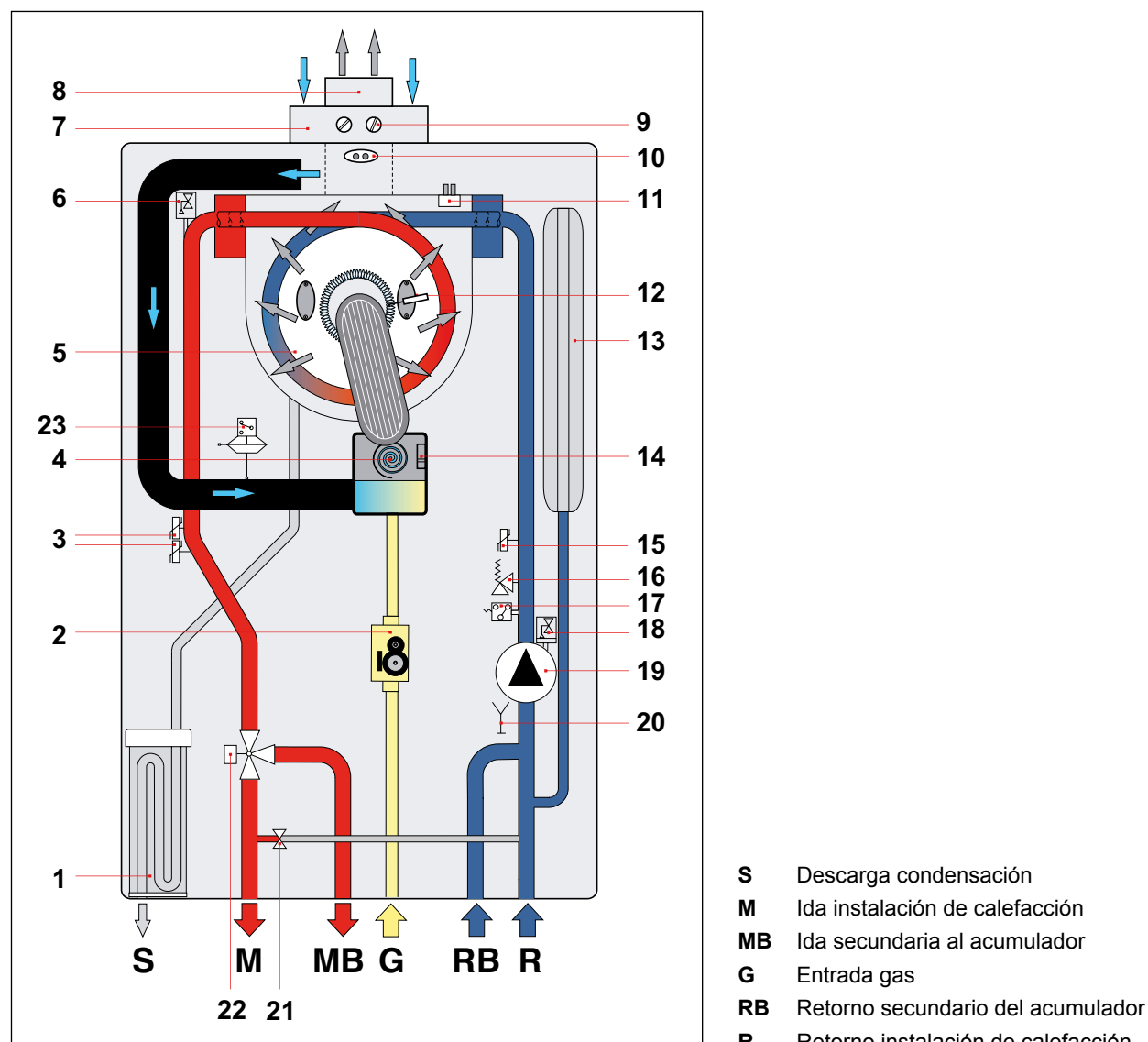
Fig. 8 Esquema hidráulico modelo KRB
