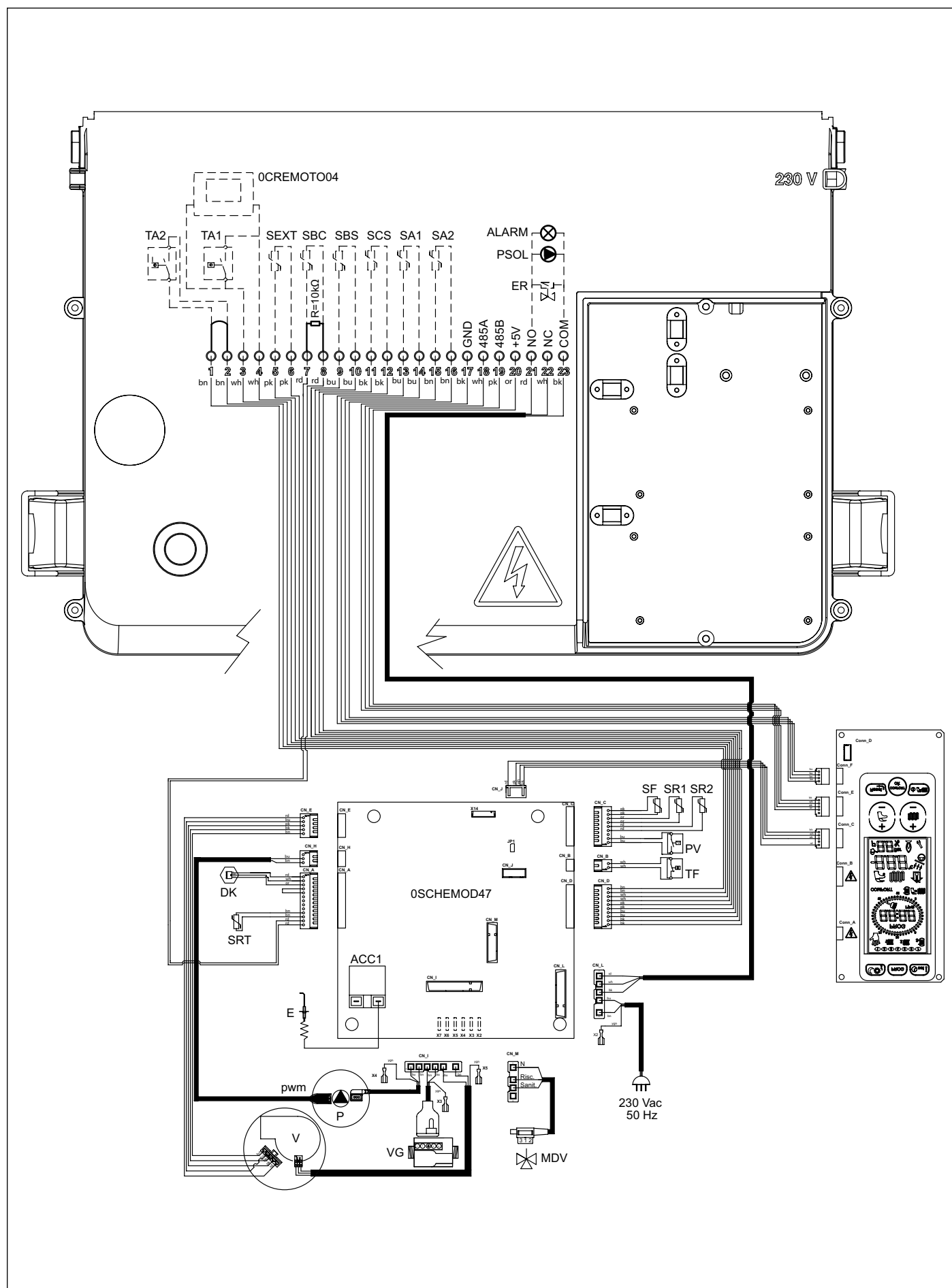
Fig. 37 Esquema eléctrico KRB
