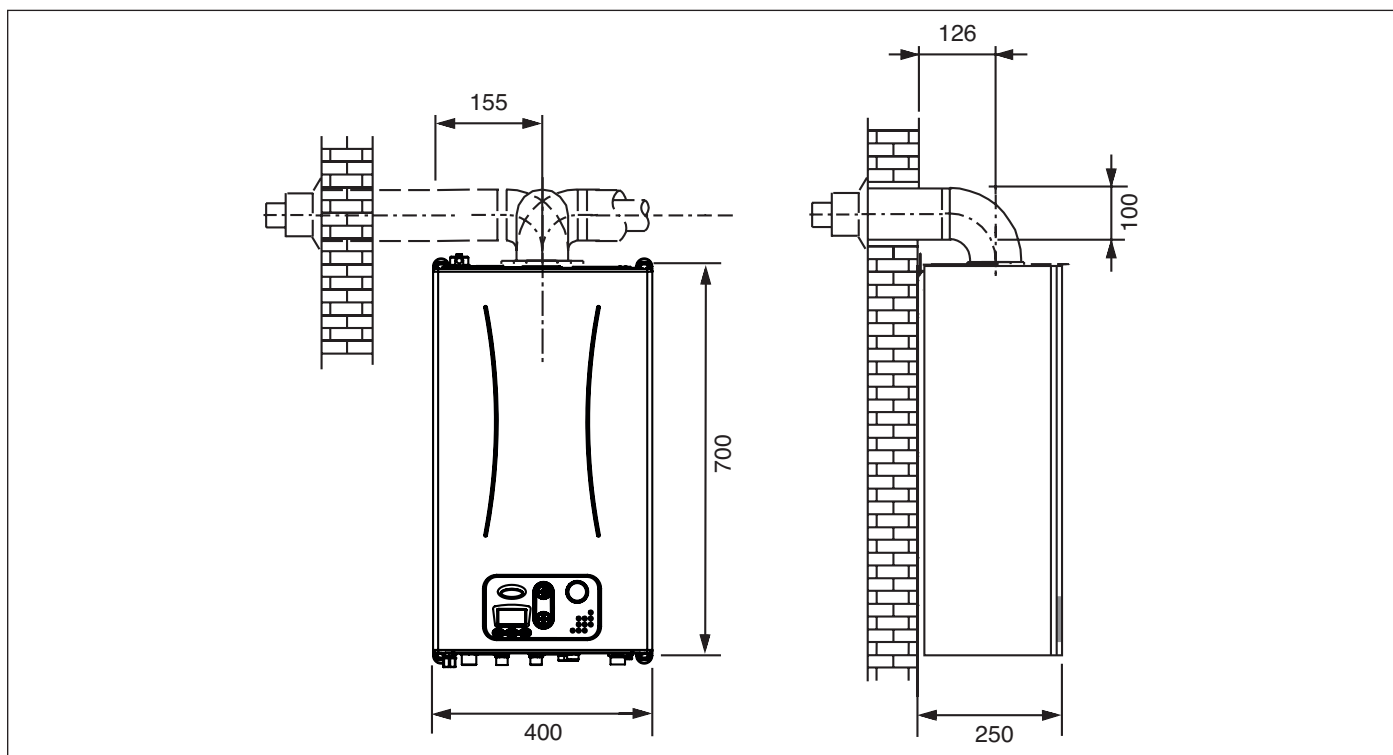
Obr. 17 Velikosti koaxiálního potrubí typ C13 - C33
