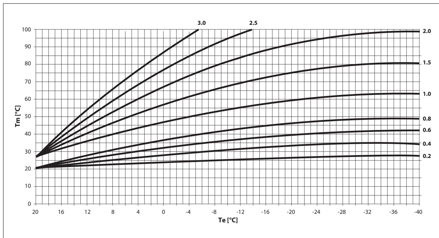
Obr. 23 Ekvitemnní křivky
