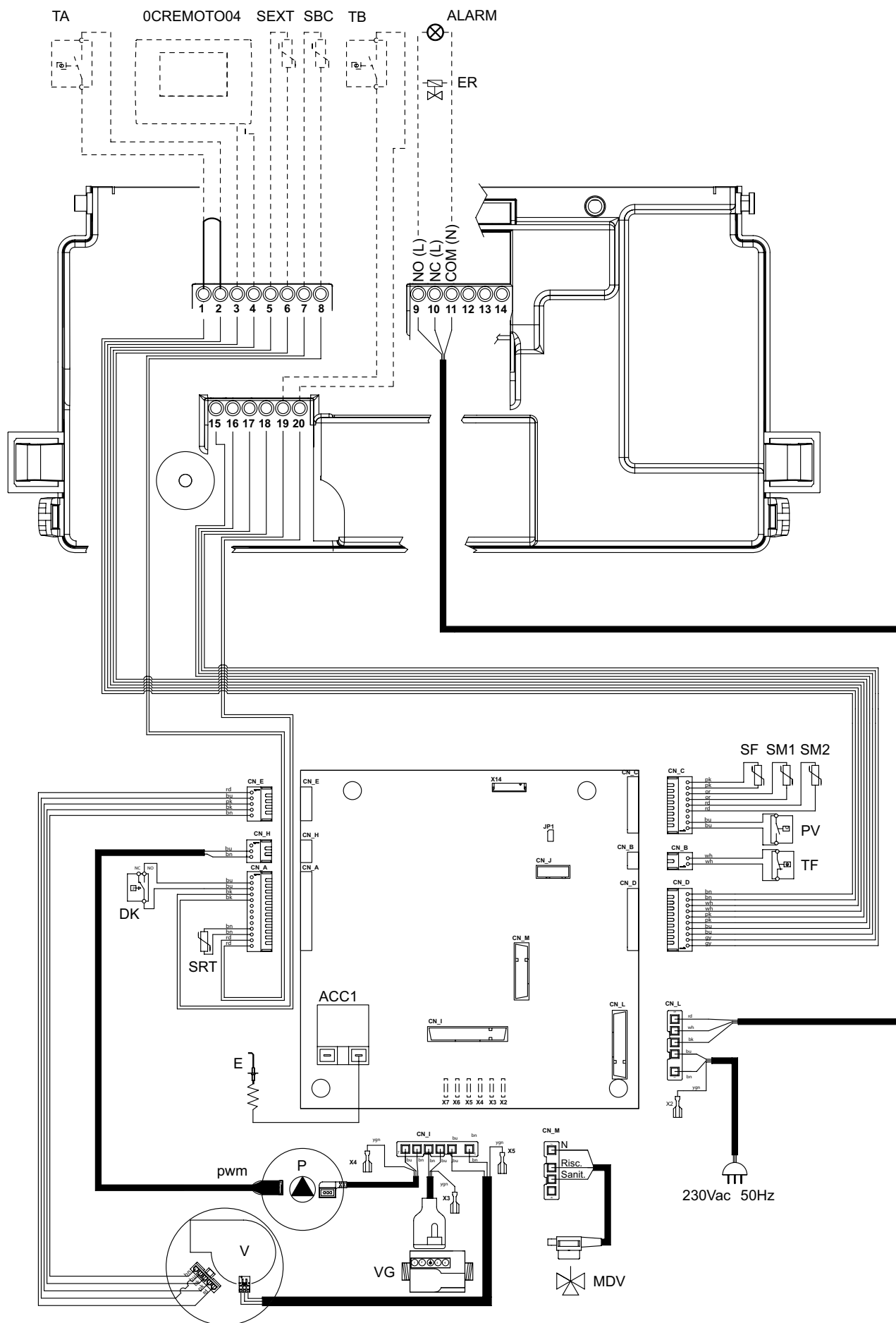
Obr. 29 Elektrické schéma KRB
