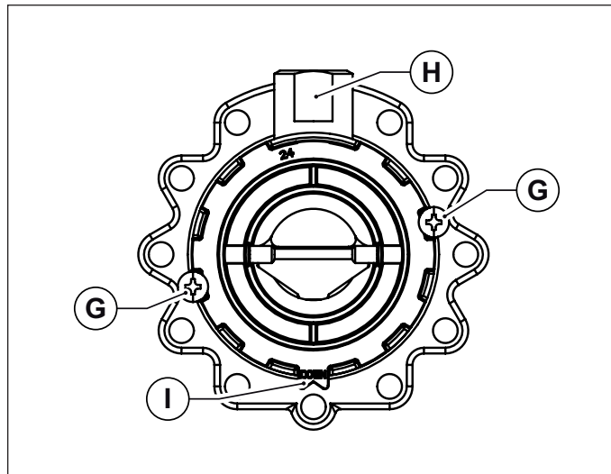
Obr. 33 Montážní orientace
