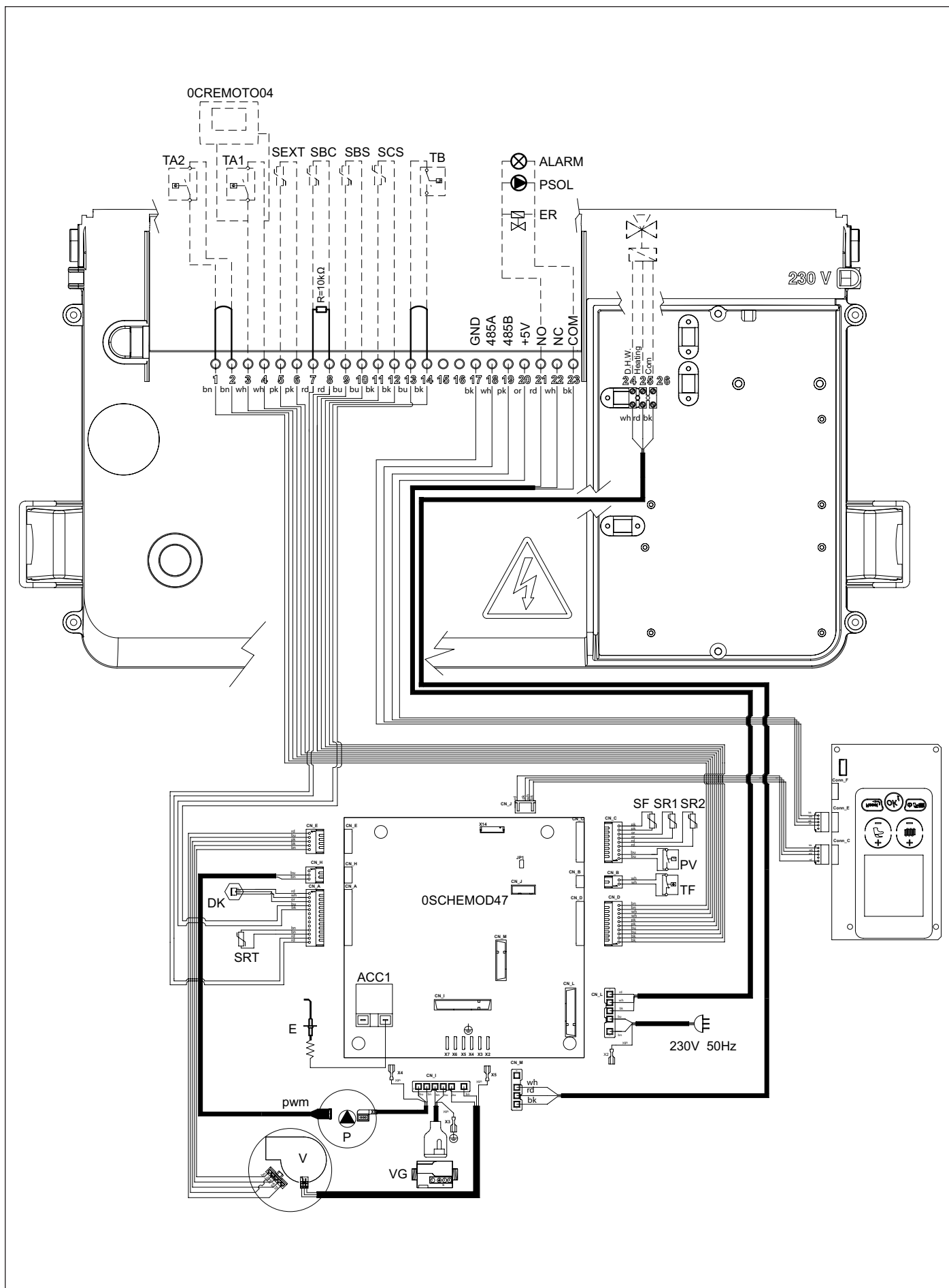
Obr. 34 Elektrické schéma model KR
