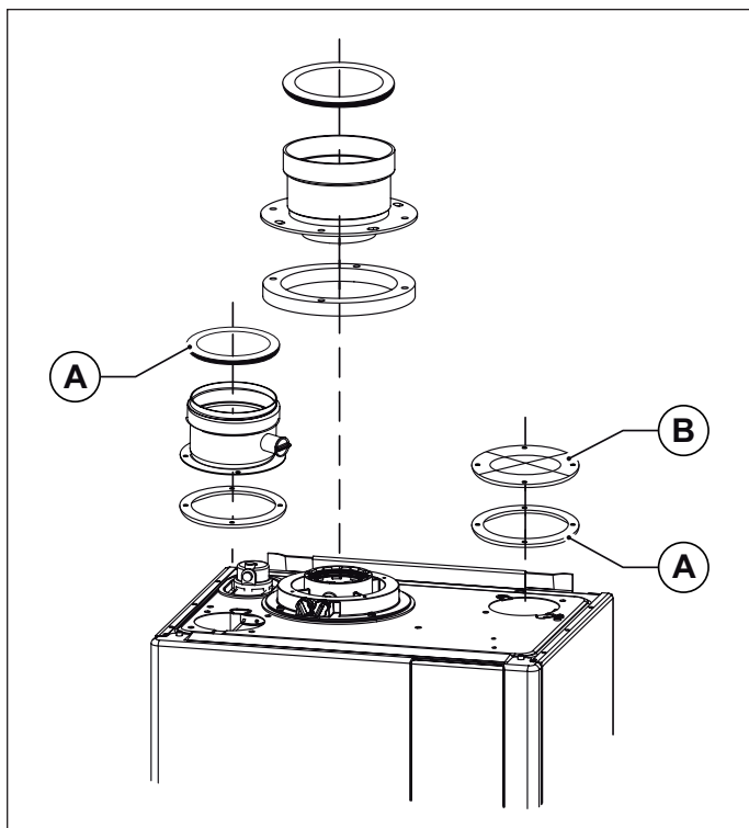
Obr. 18 Koaxiální potrubí typu C43 - C53 - C83
