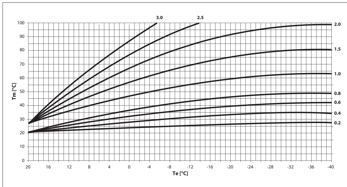
Obr. 24 Ekvitermní křivky
