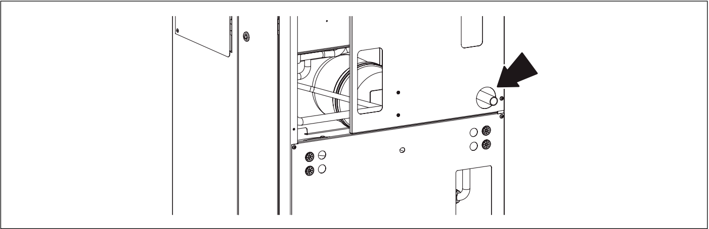
Abb. 20 Abgas-Kondensatableitung
