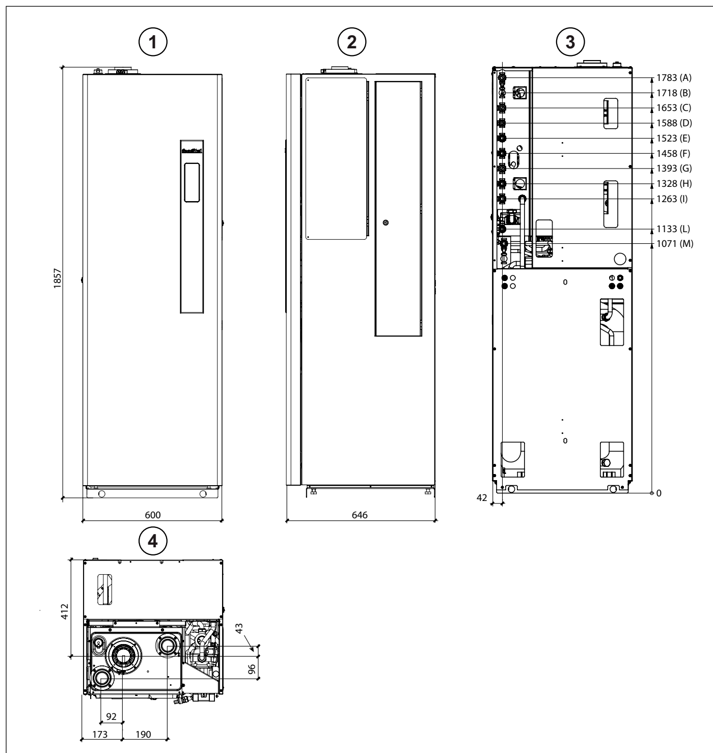
rys. 3 Wymiary
