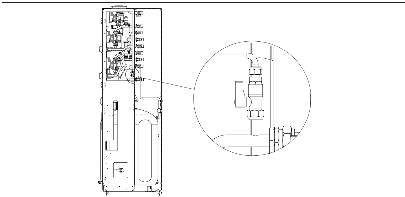
rys. 2 Zawór napełniający
