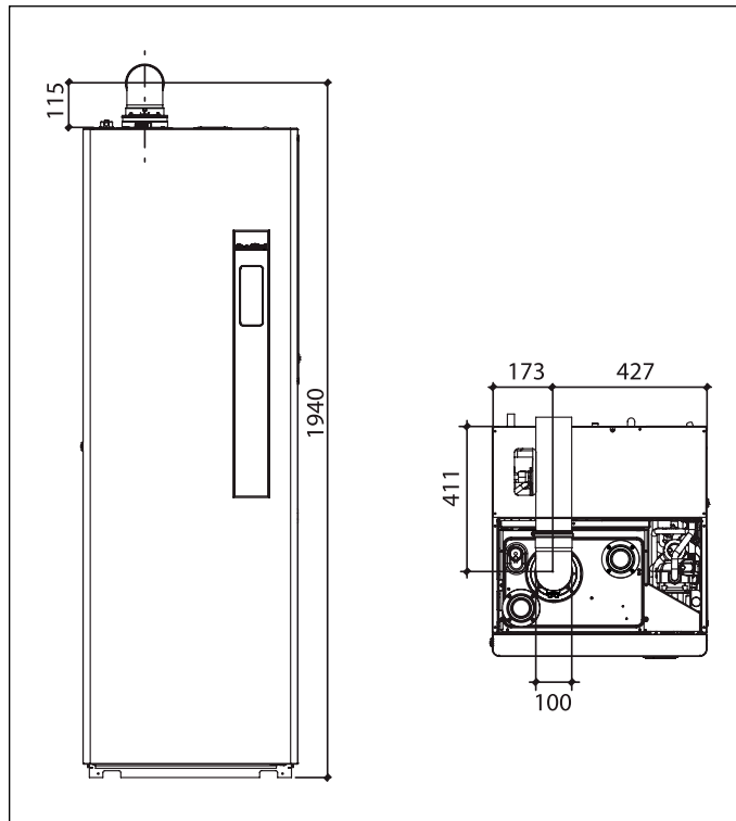
rys. 17 Wymiary przewodów koncentrycznych typu C33
