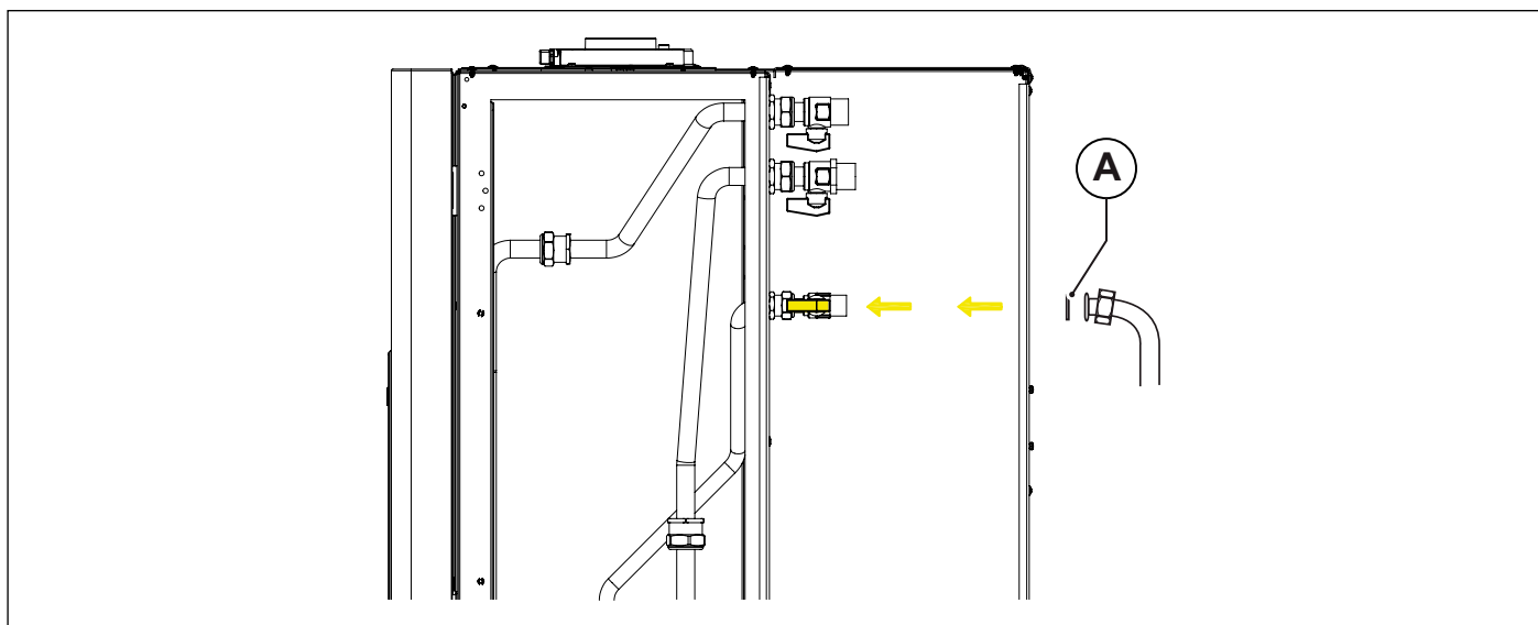
rys. 22 Podłączenie do sieci gazowej
