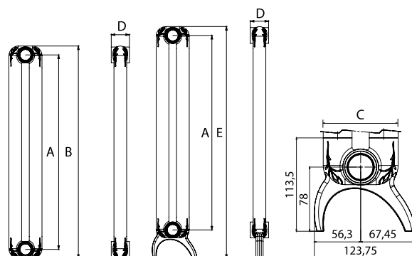
ROZMĚRY VYJÁDRĚNÉ V MILIMETRECH
