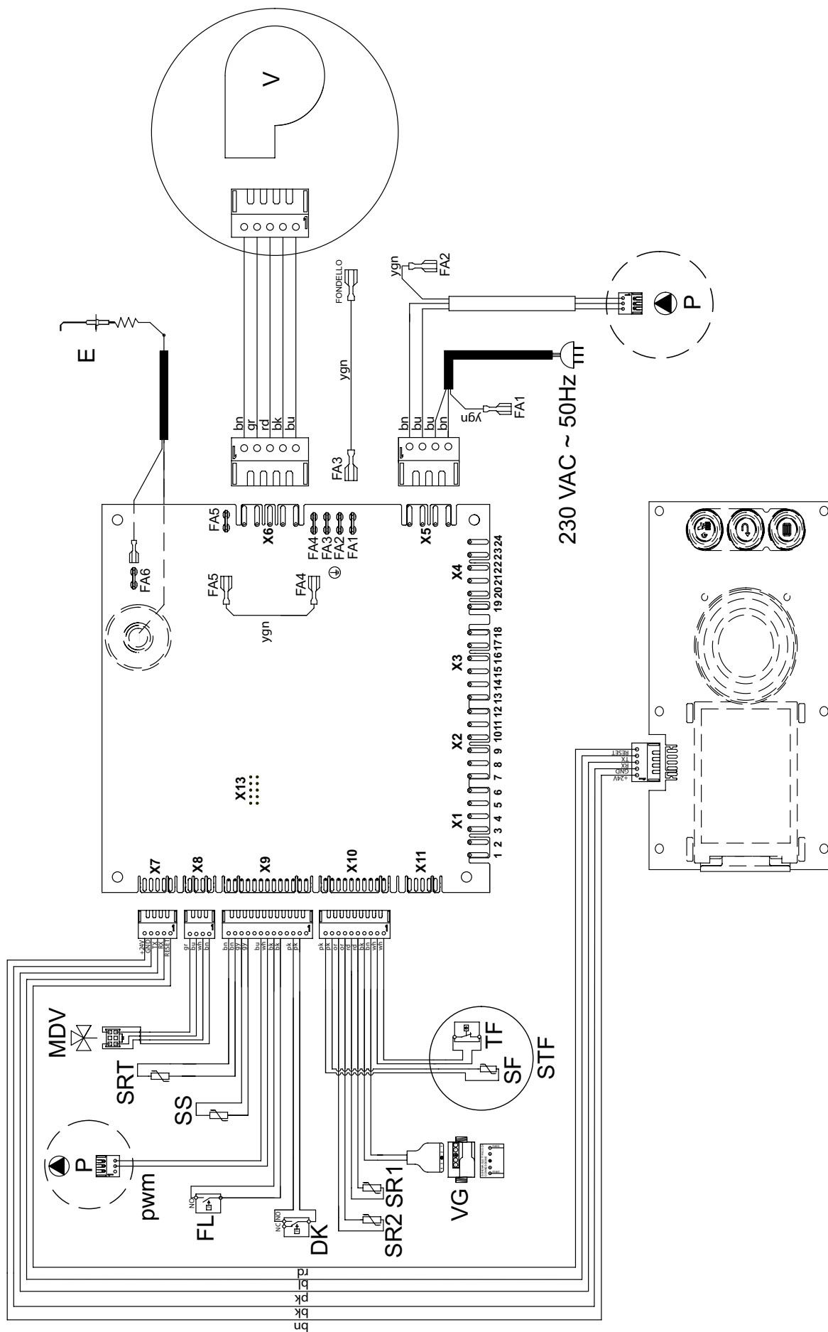
Рис. 19 Електрична схема КС (II)
