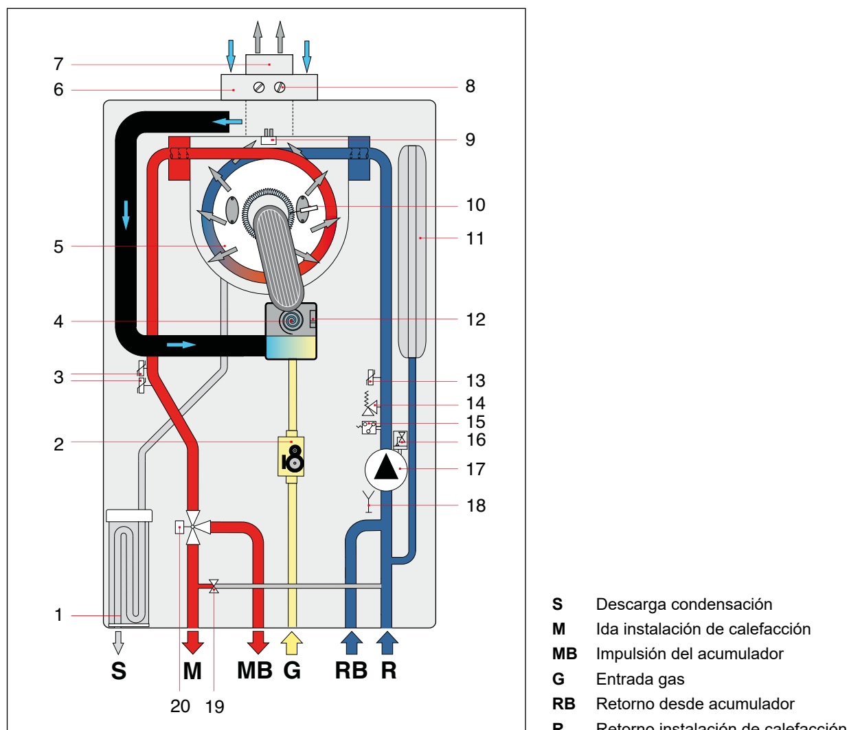
Fig. 6 Esquema hidráulico KRB
