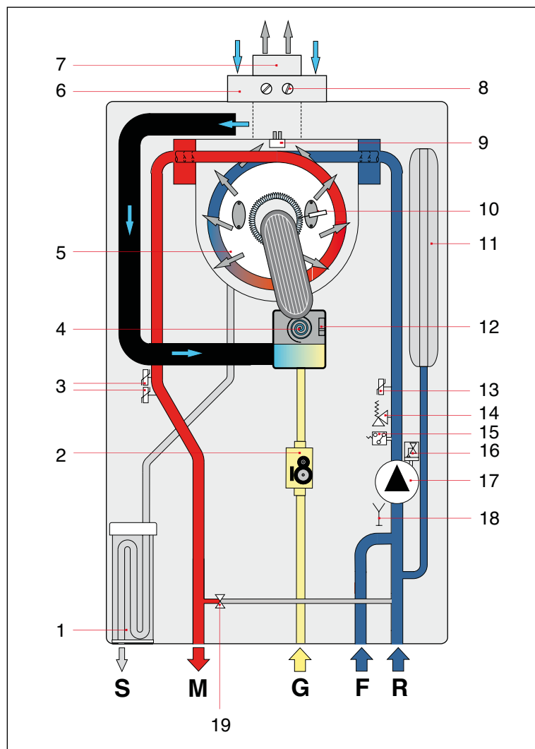
Fig. 5 Esquema hidráulico KR
