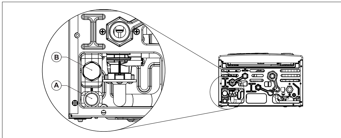
Fig. 21 Evacuare condens
