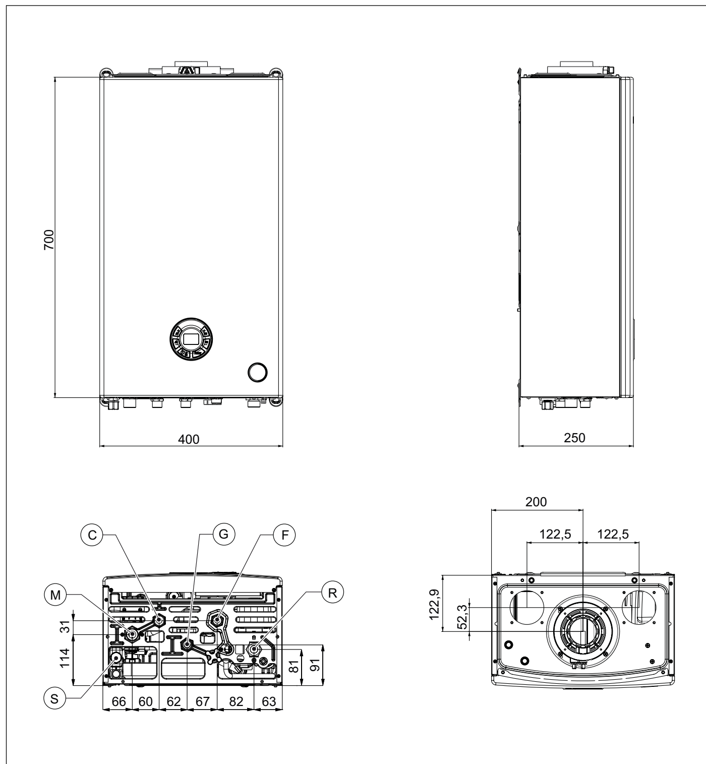
Fig. 3 Dimensiuni
