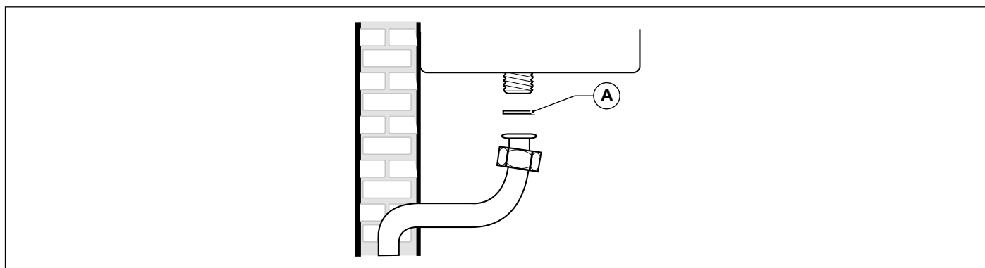
Fig. 20 Racordare la rețeaua de gaz
