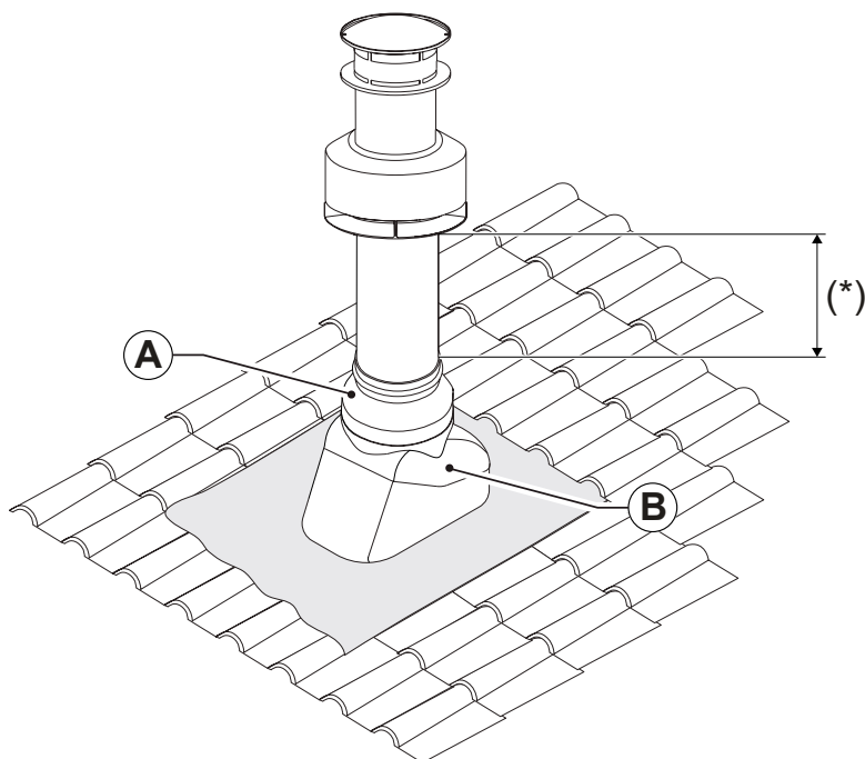
Fig. 16 Instalarea coșului de fum pe acoperiș
