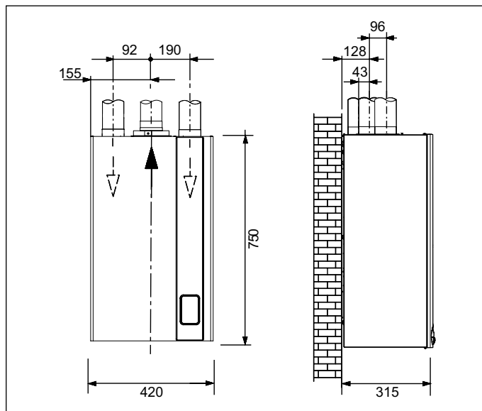
Fig. 19 Dimensiuni conducte coaxiale tip C43 – C53 – C83
