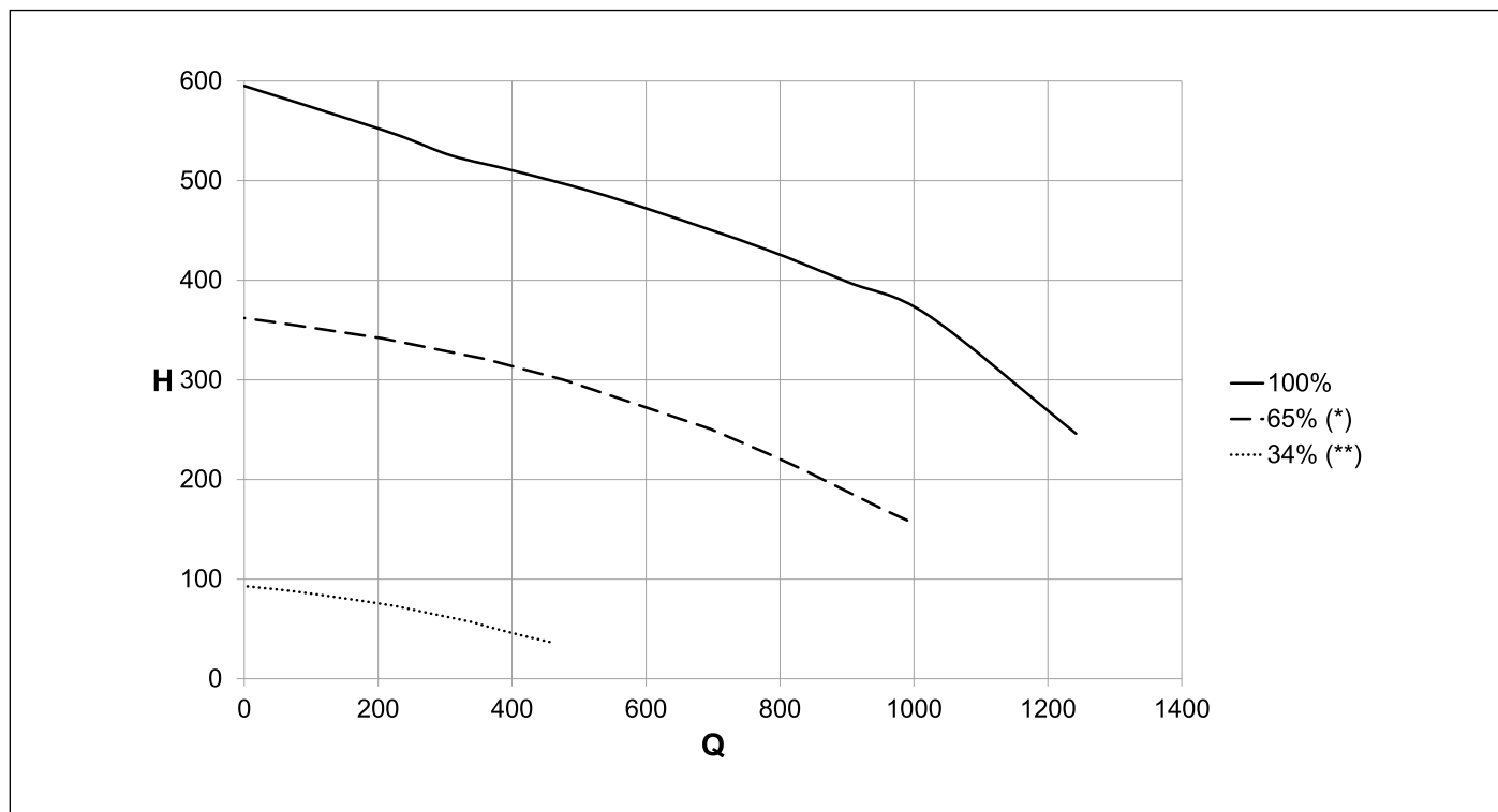
Fig. 28 Presiune disponibilă KC-KR-KRB 32
