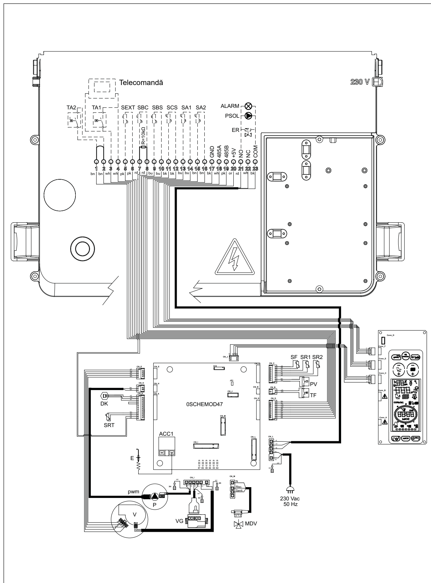
Fig. 37 Schema electrică KRB
