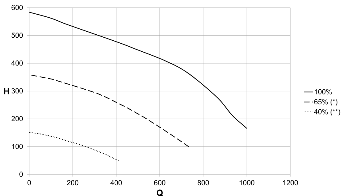
Fig. 25 Presiune disponibilă KC-KR-KRB 12
