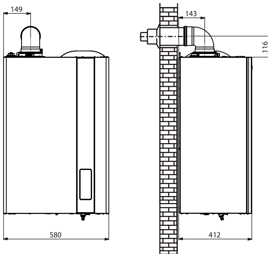
Fig. 16 Dimensiuni conducte coaxiale tip C13 - C33
