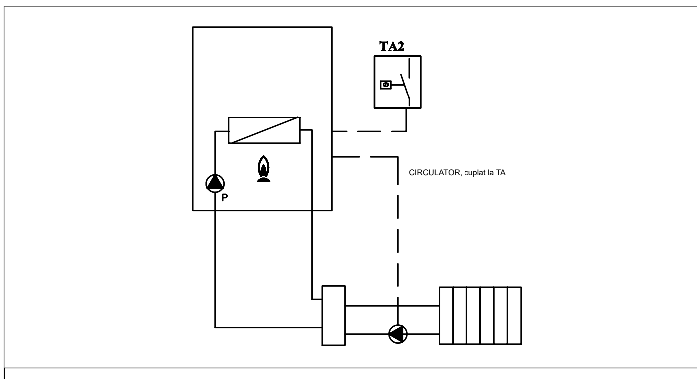
Fig. 30 Releu cu solicitare (P17=3)
