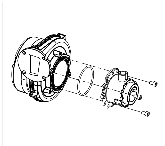
Fig. 33 Amestecător
