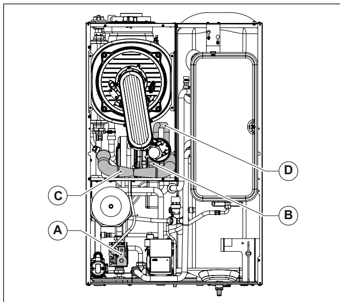
Fig. 32 Tobă de aspirație
