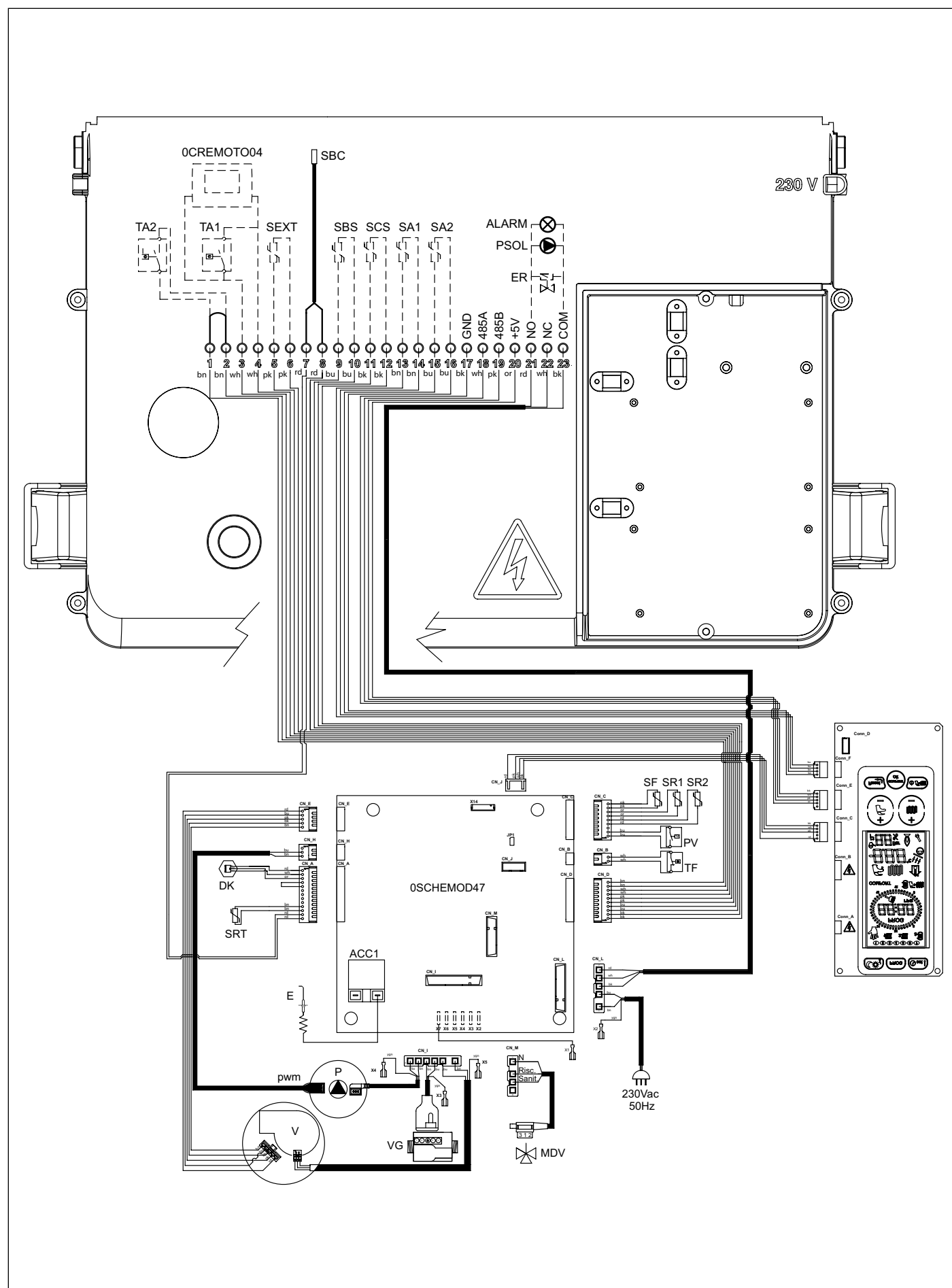
Fig. 25 Schema electrică
