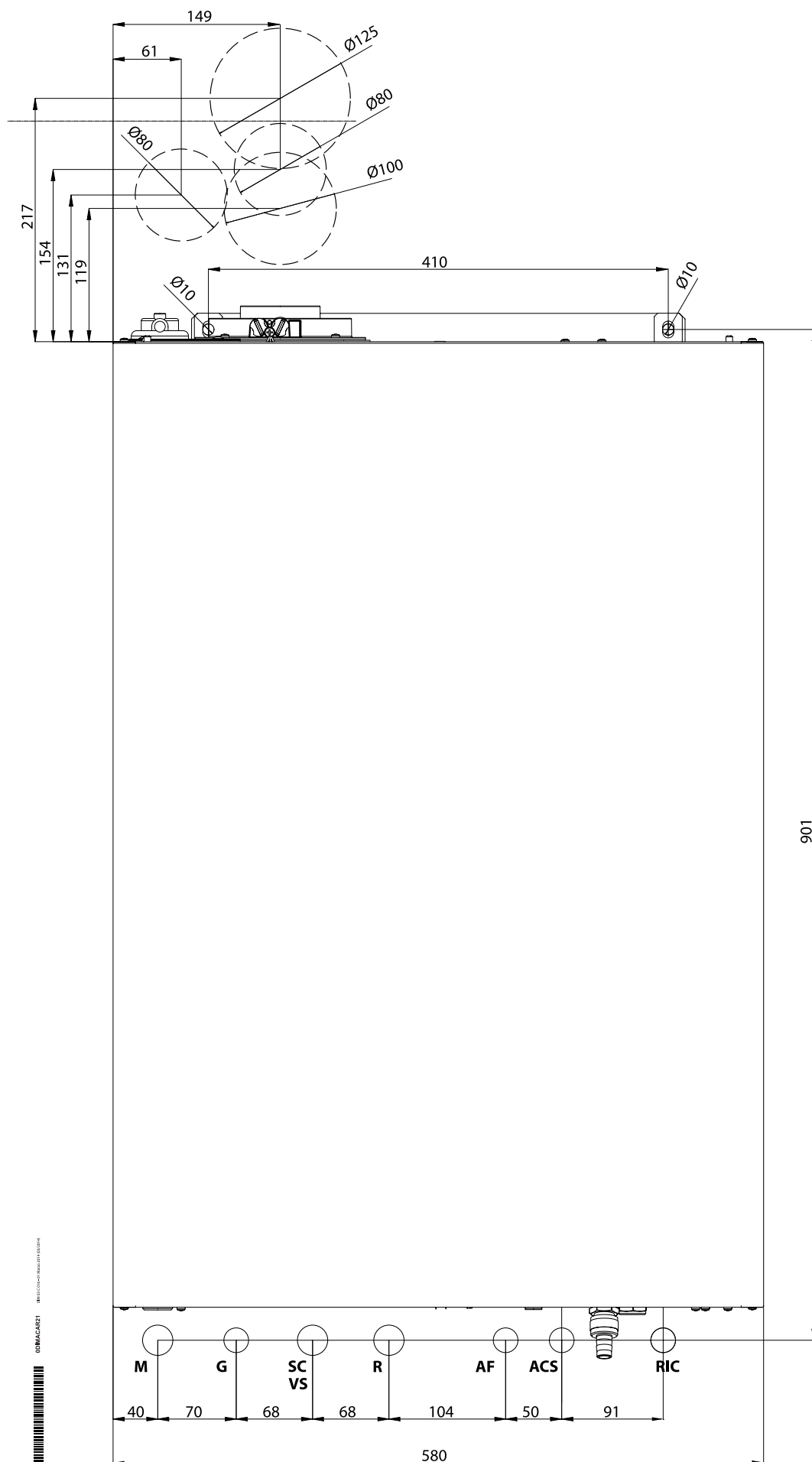
Fig. 6 Șablon de hârtie
