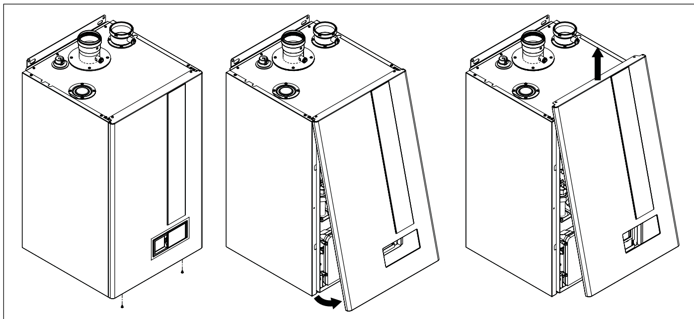
Fig. 40 Deschidere carcasă
