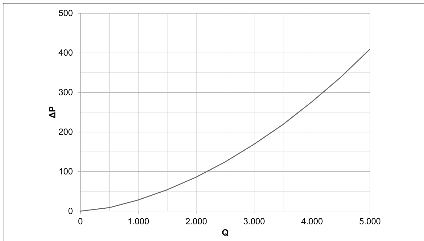
Fig. 25 Rezistență hidraulică KR 99 - KR 120
