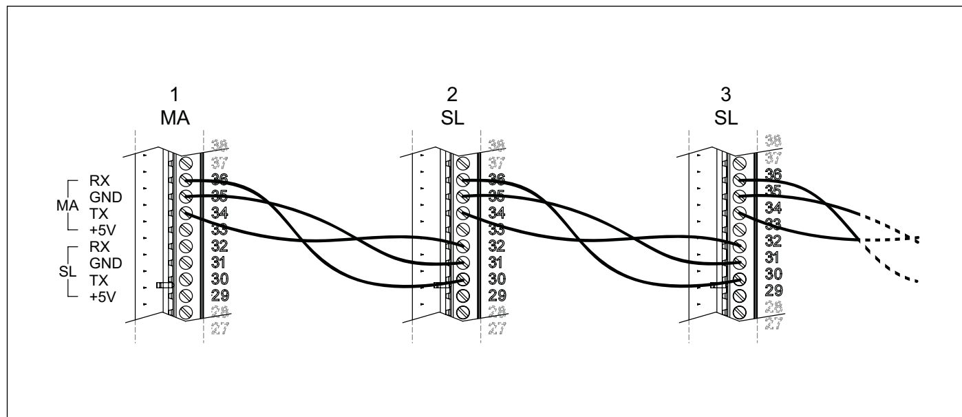
Fig. 39 Conectare în cascadă
