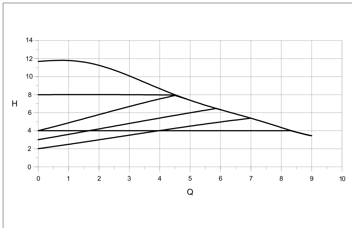
Fig. 32 Presiune disponibilă UPMXXL 25 - 120 - 180 AUTO
