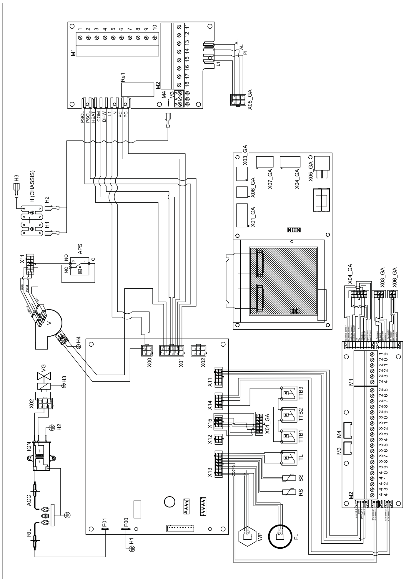
Fig. 37 Schema electrică KR 150
