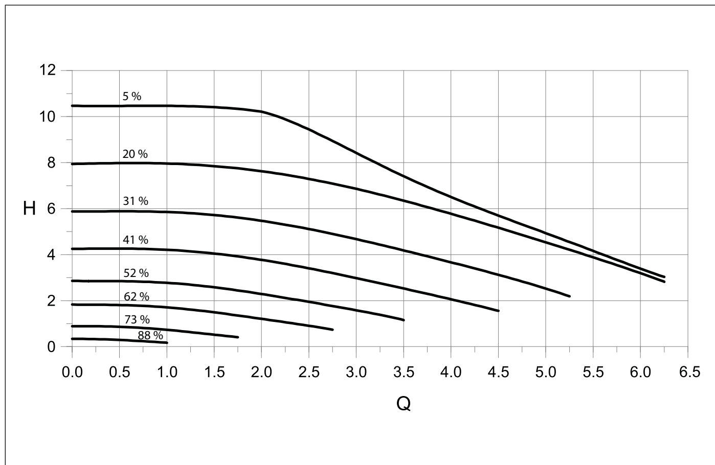
Fig. 30 Presiune disponibilă UPML 25 - 105 - 180 PWM
