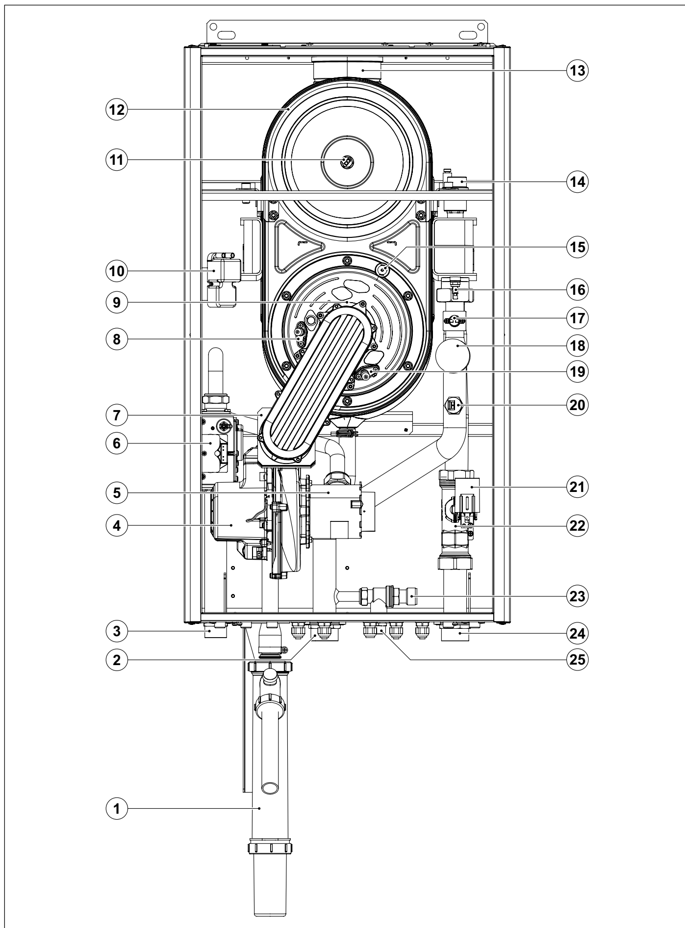
Fig. 7 Componente KR 99 - KR 120 (I)
