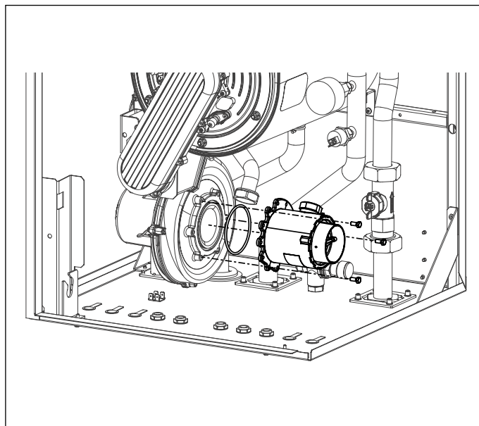
Fig. 42 Amestecător
