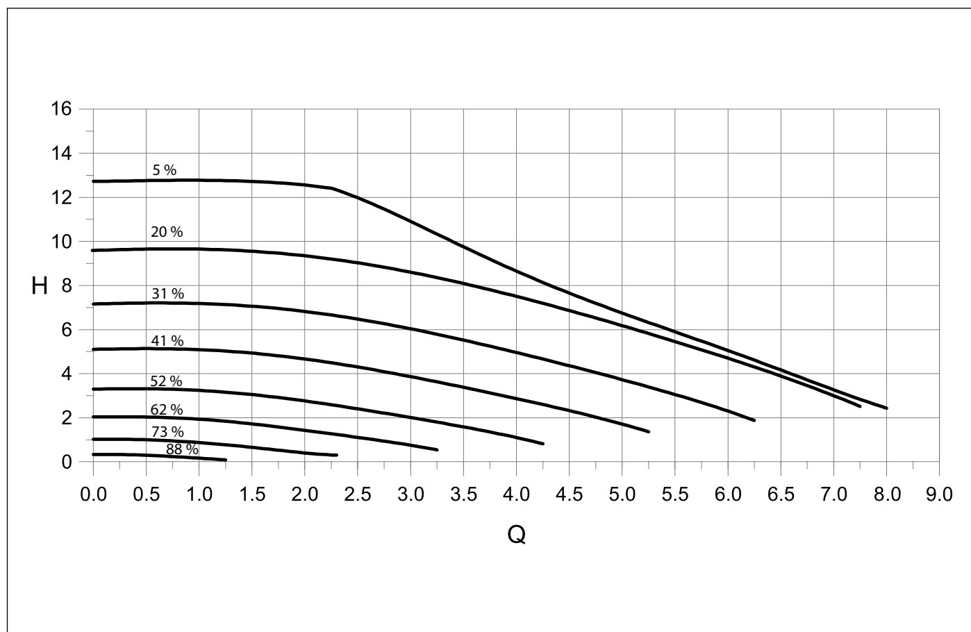
Fig. 31 Presiune disponibilă UPMXL 25 - 125 - 180 PWM
