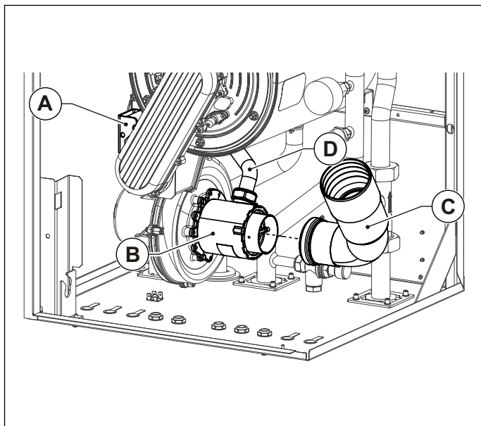
Fig. 41 Tobă de aspirație
