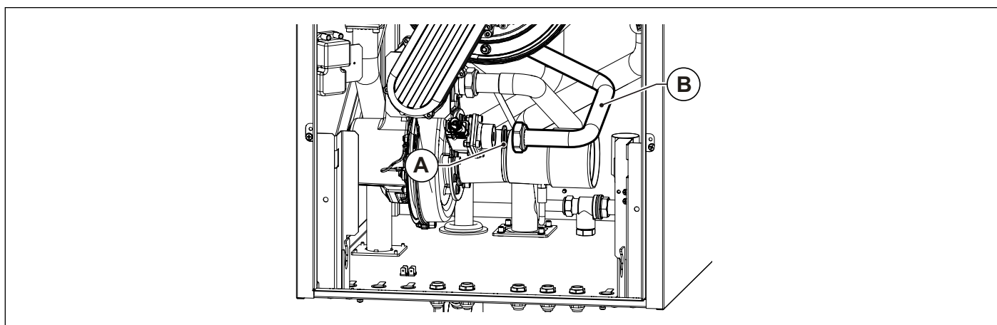
Fig. 46 Înlocuirea diafragmei de gaz KR 150
