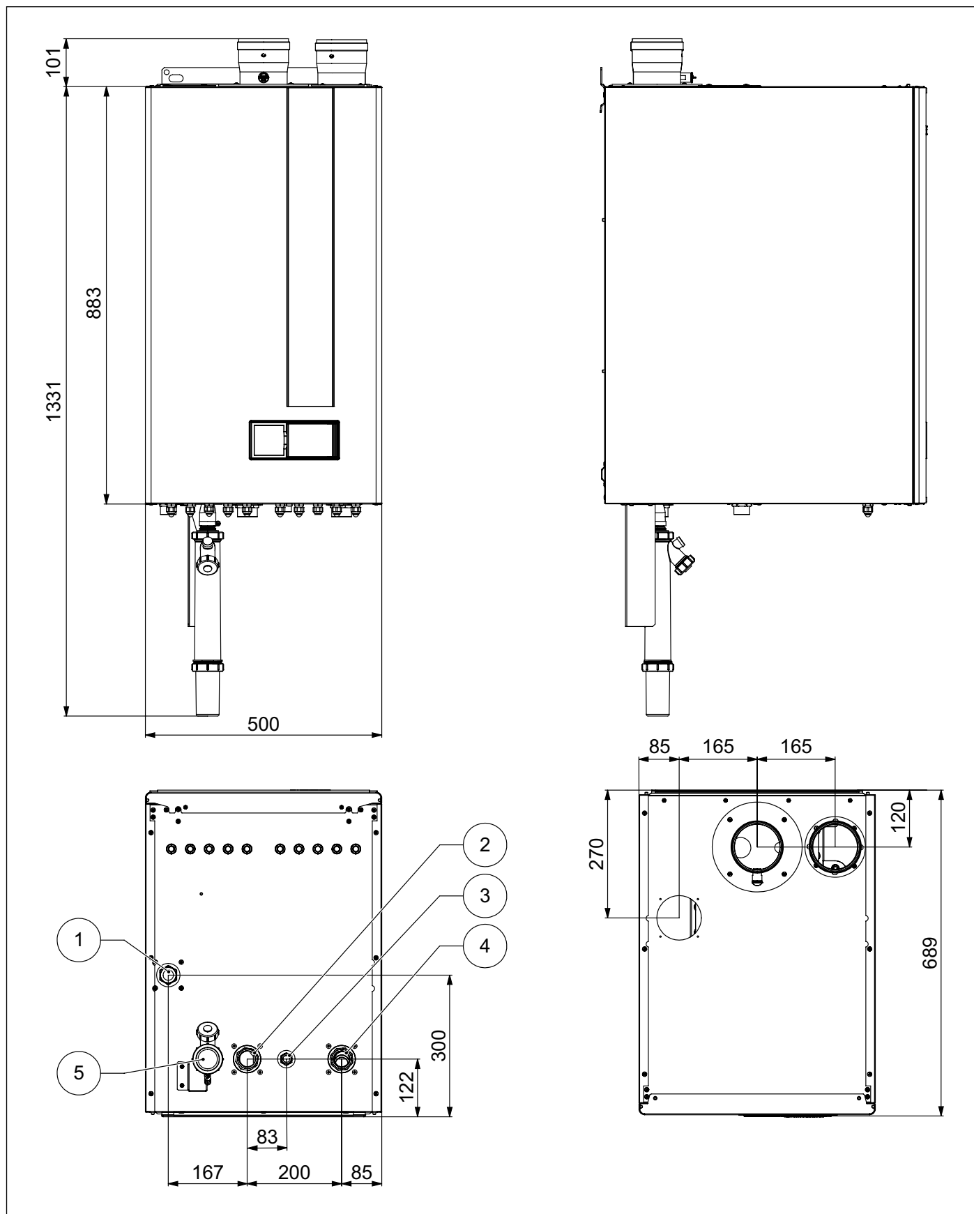
Fig. 4 Dimensiuni KR 99 - KR 120 - KR 150
