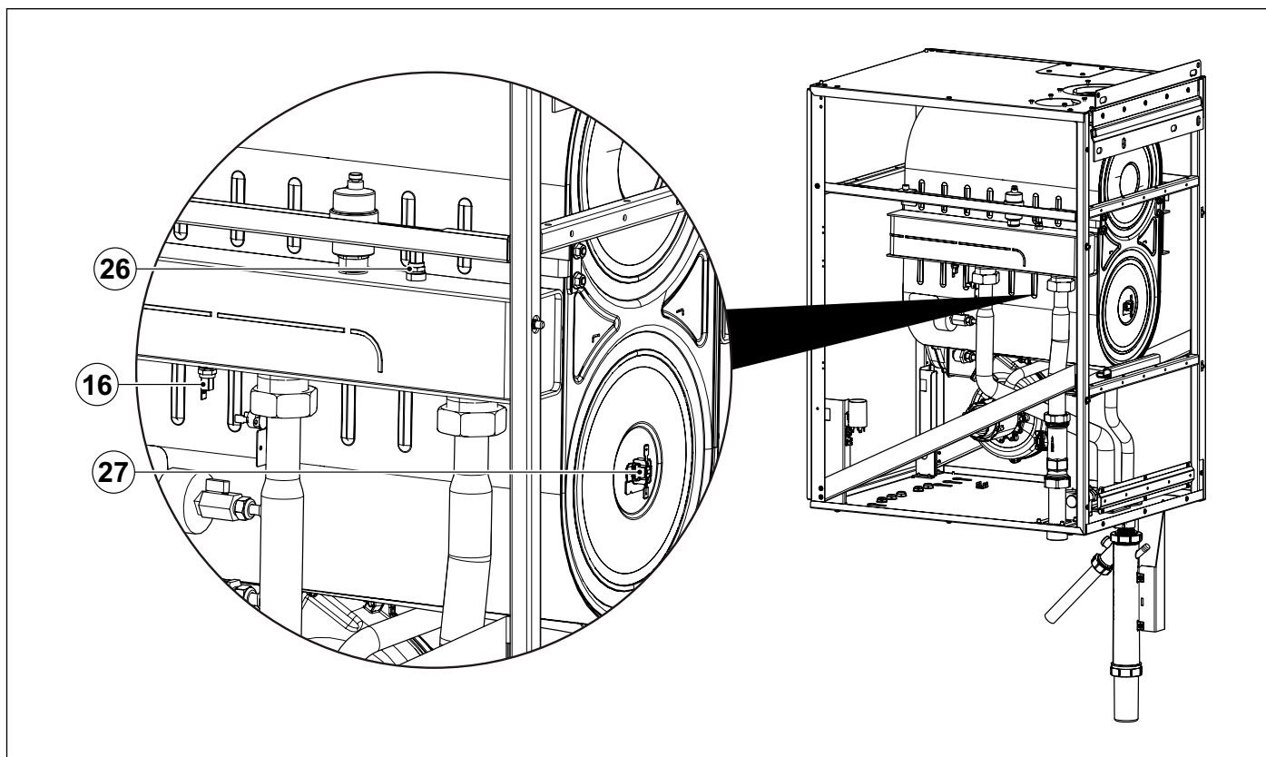
Fig. 8 Componente KR 99 - KR 120 (II)
