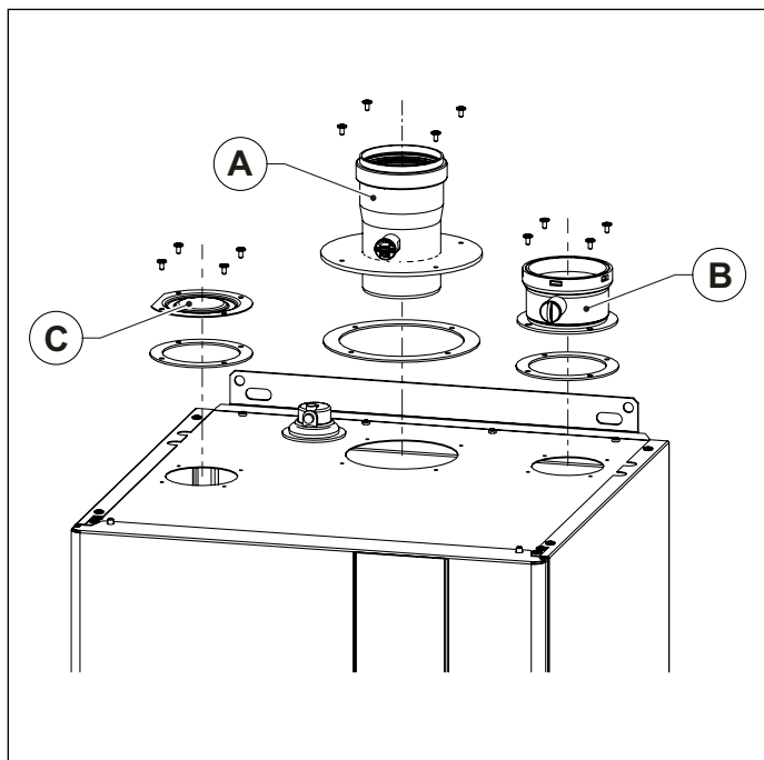
Fig. 11 Instalarea kit-ului pentru conducte duble
