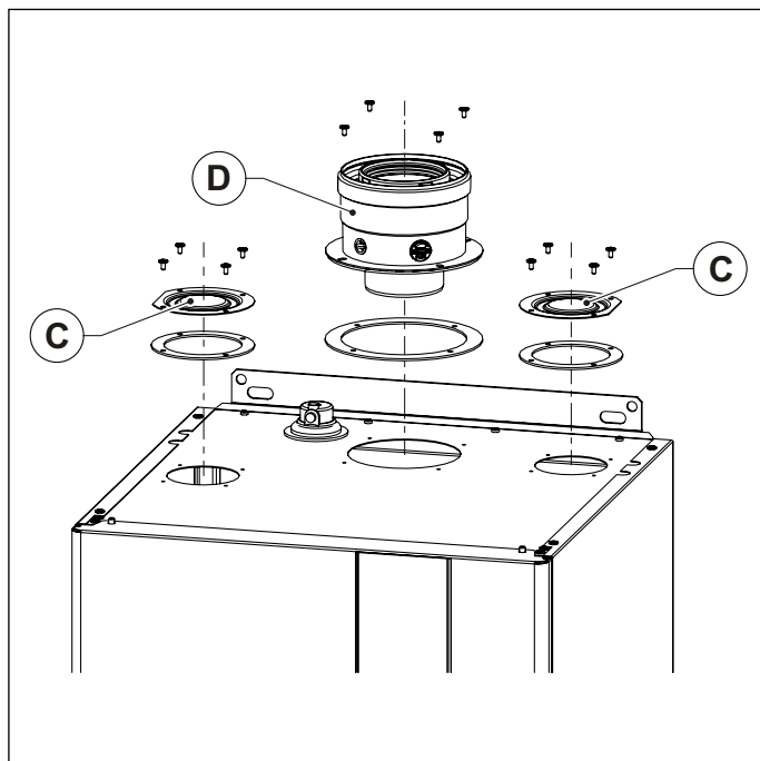
Fig. 12 Instalarea kit-ului pentru conducte coaxiale
