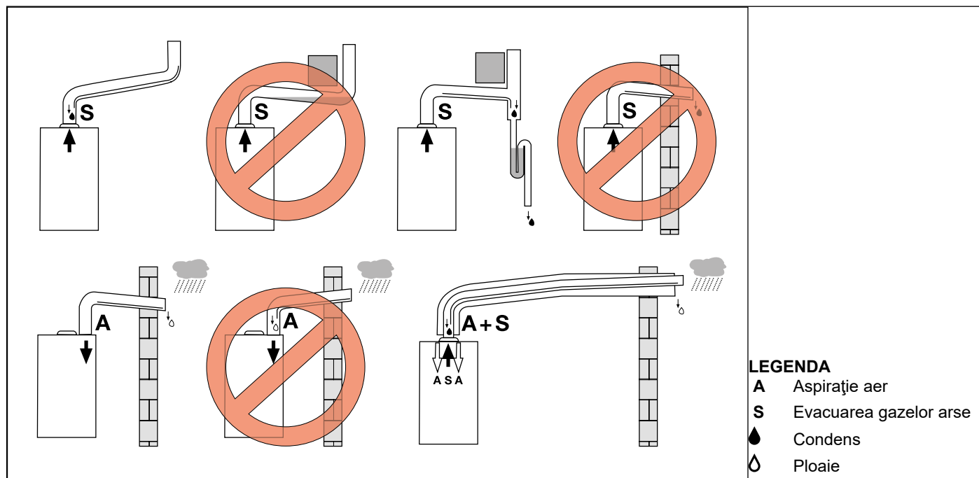
Fig. 13 Exemple de instalare
