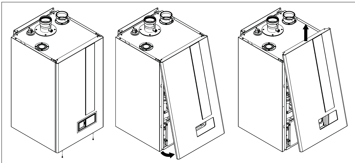
Fig. 31 Deschidere carcasă
