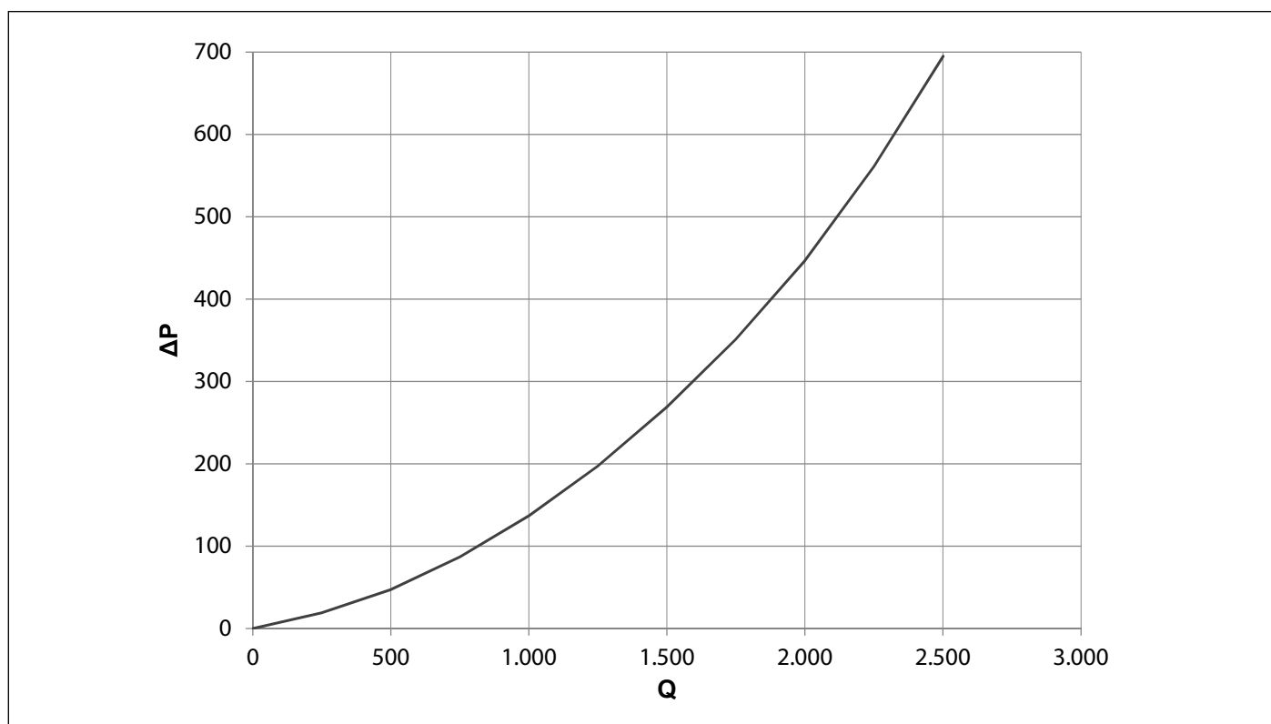
Fig. 21 Rezistență hidraulică KR 45
