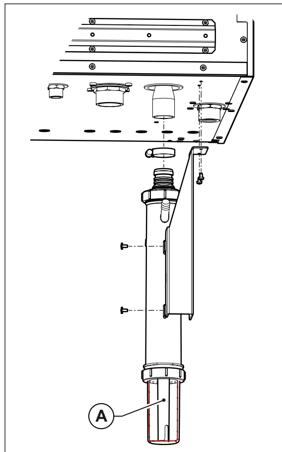
Fig. 10 Fixarea sifonului
