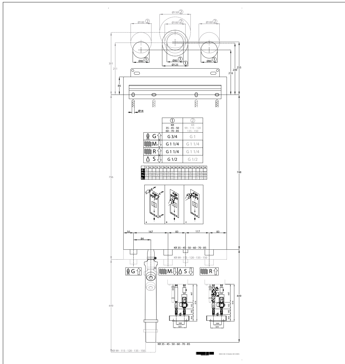
Fig. 9 Șablon de hârtie
