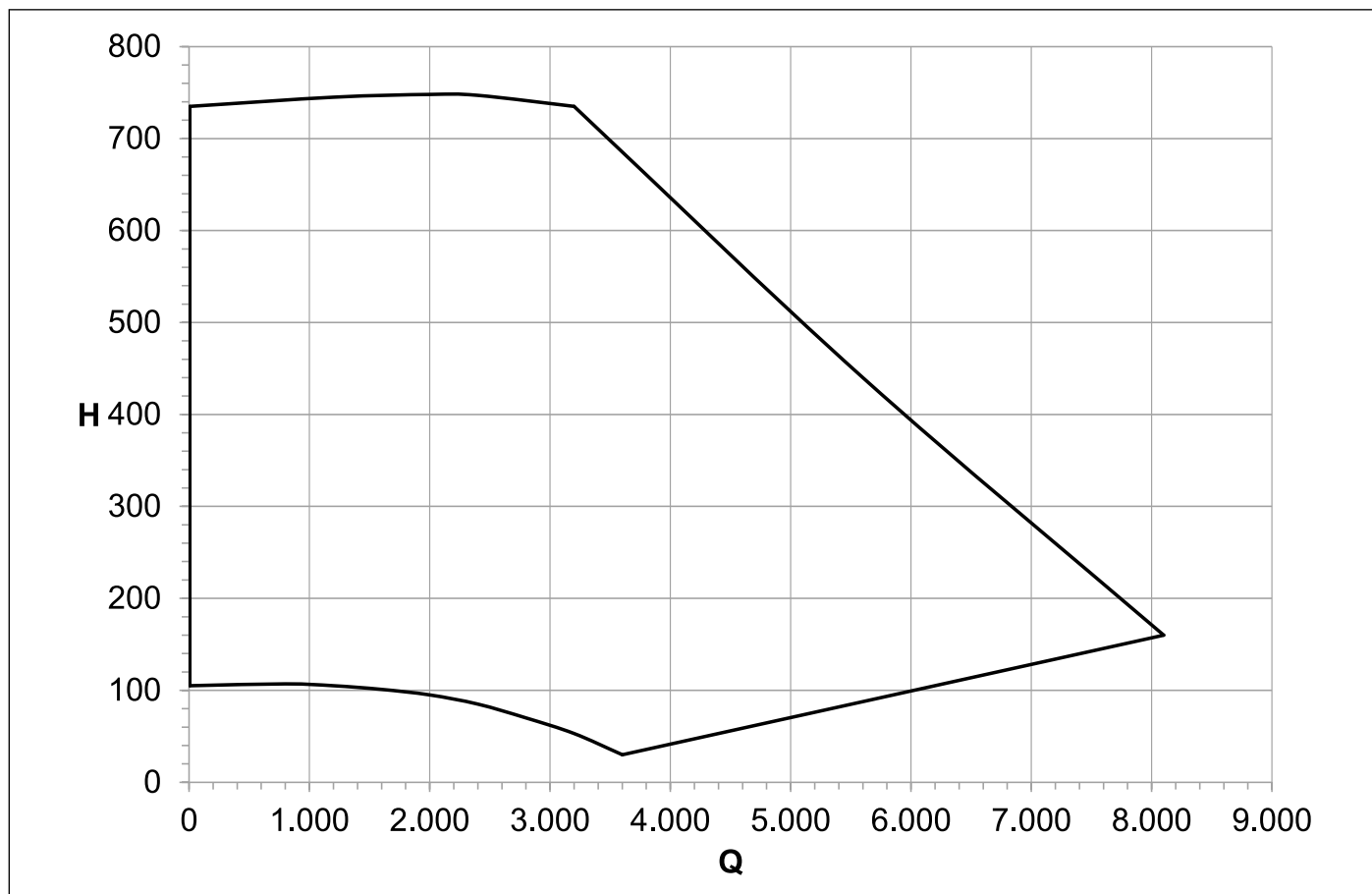
Fig. 24 Presiune disponibilă YONOS PARA HF 25/7
