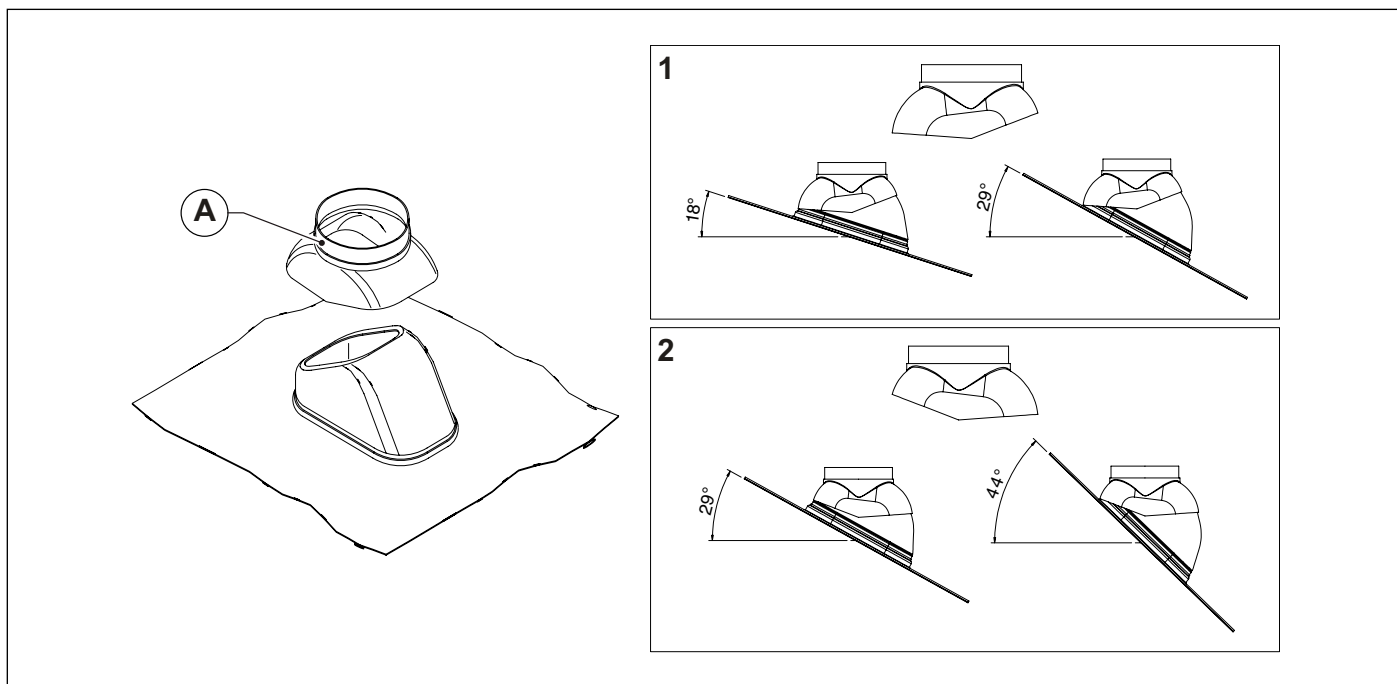
Fig. 16 Placă pentru acoperișuri înclinate
