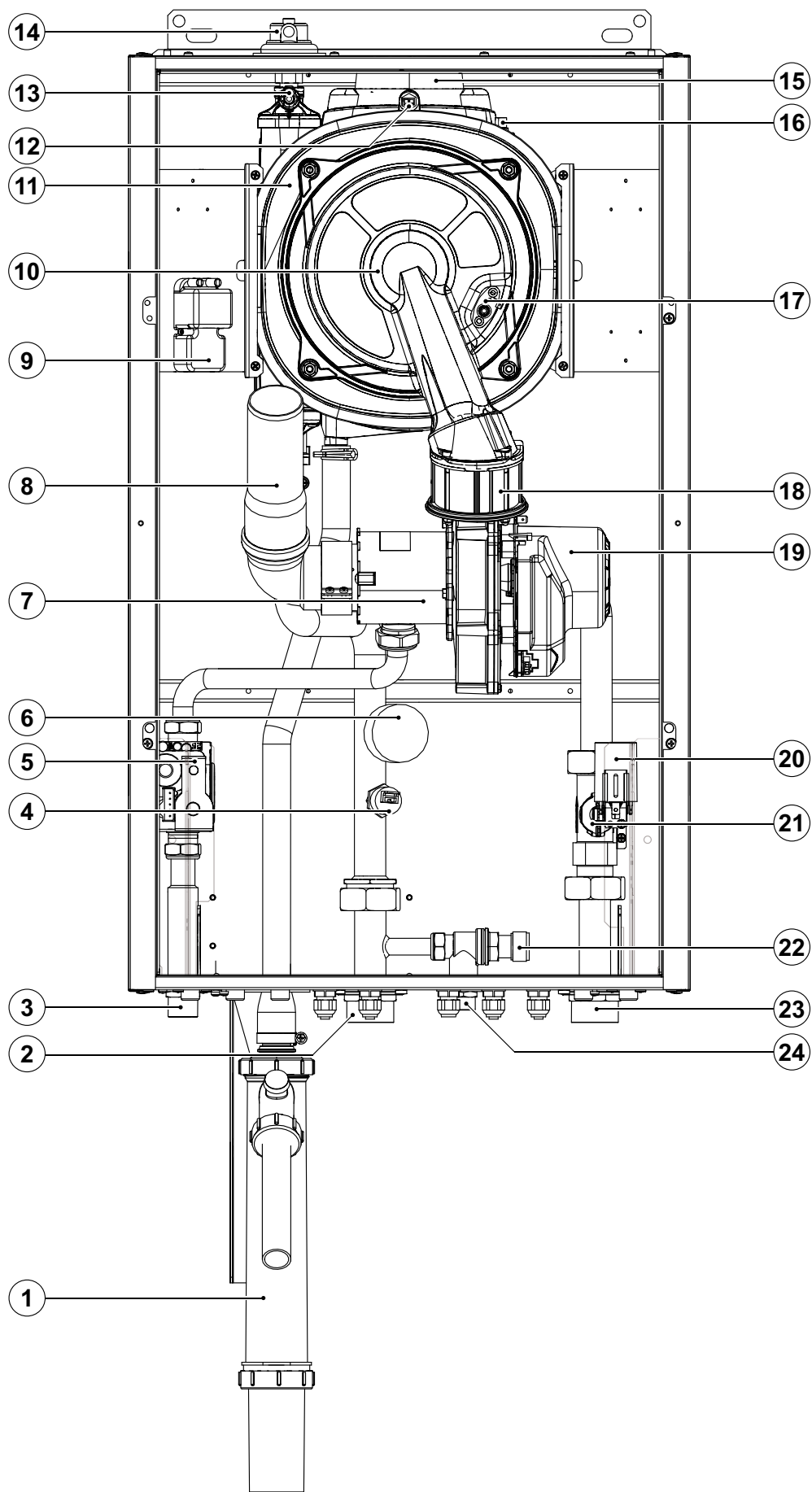
Fig. 6 Componente KR 60 (I)
