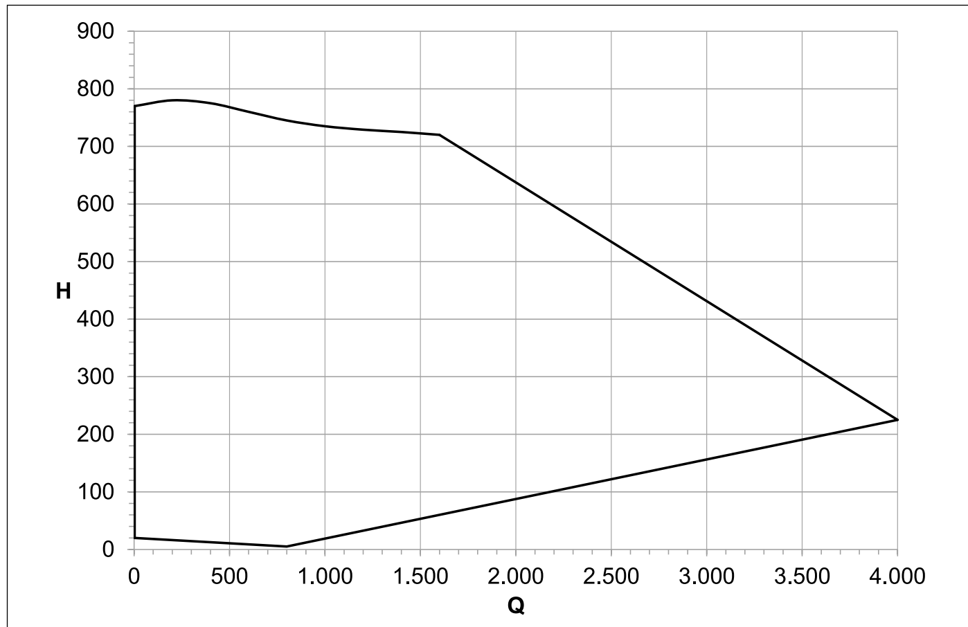
Fig. 23 Presiune disponibilă YONOS PARA RS 25/7.5
