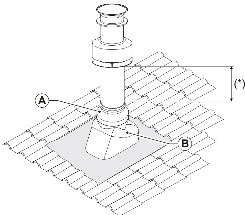
Fig. 17 Instalarea coșului de fum pe acoperiș
