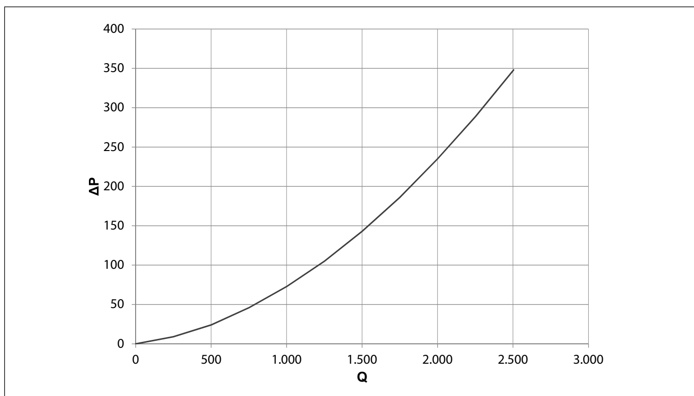
Fig. 22 Rezistență hidraulică KR 60
