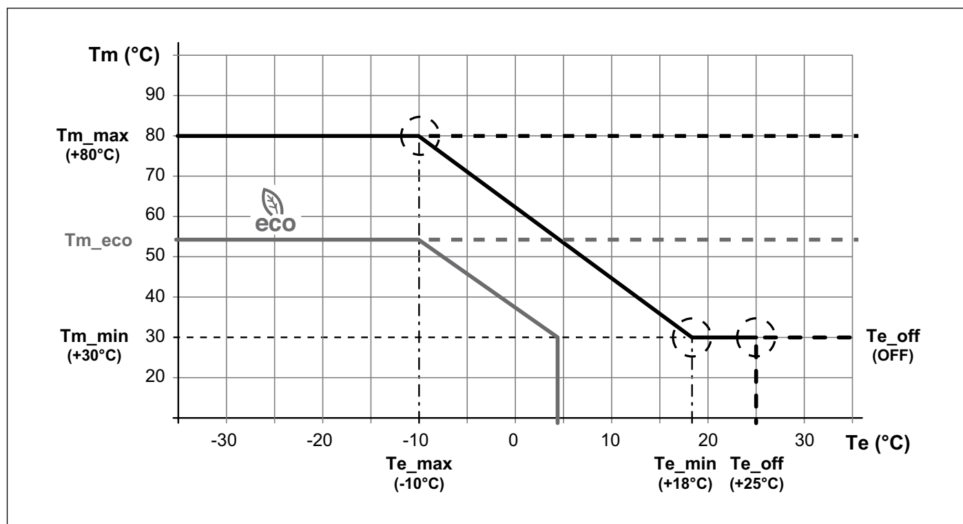
Fig. 19 Curbă climatică
