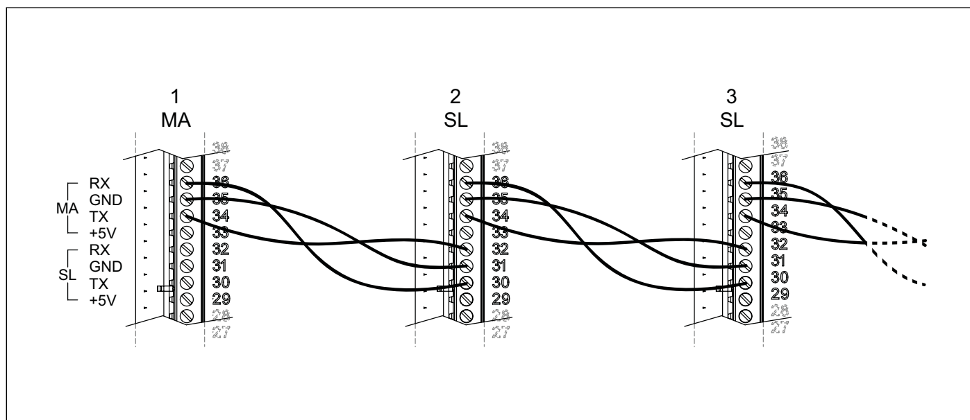
Fig. 30 Conectare în cascadă
