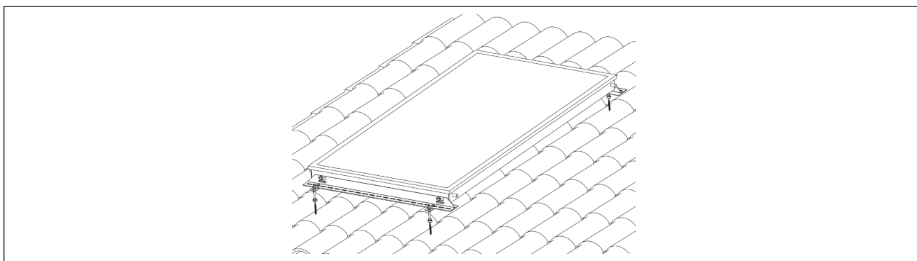
fig. 10 - Installazione su tetto inclinato attraverso tegola o coppo
